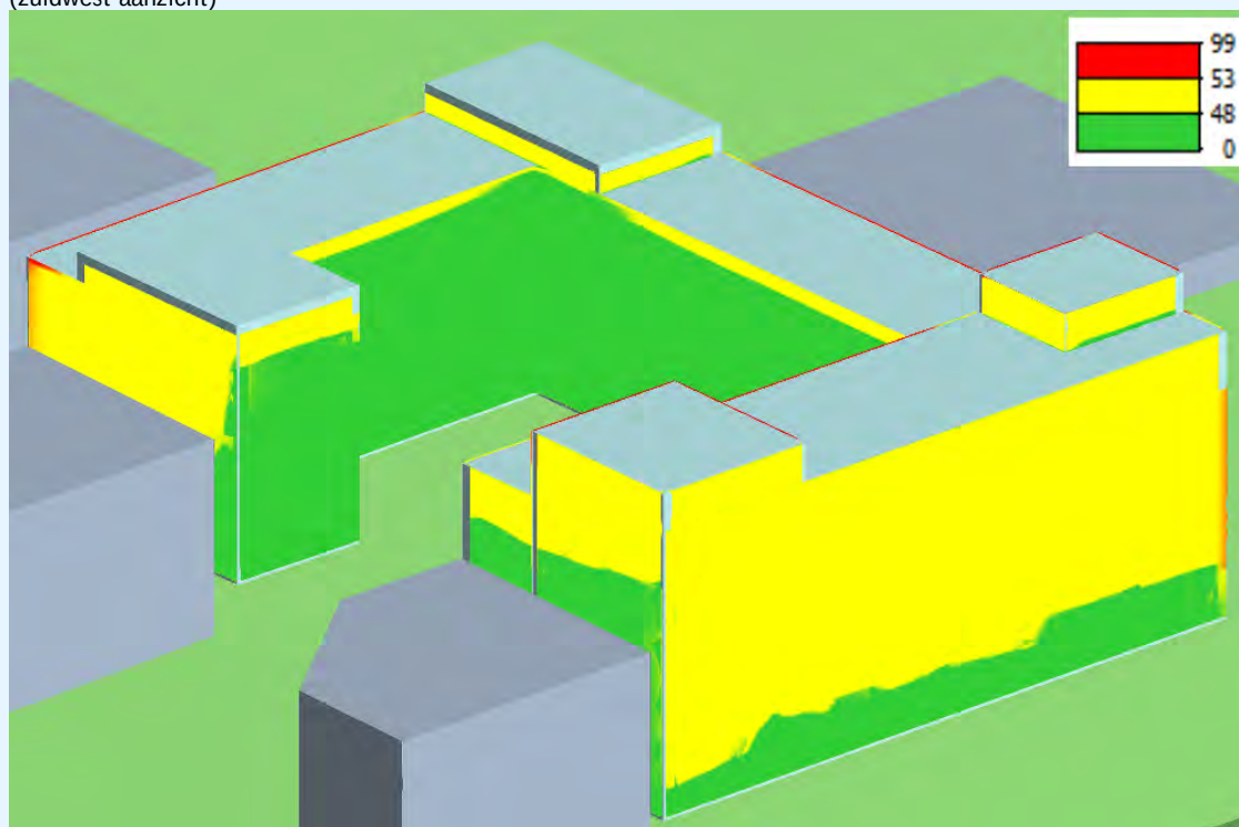
figuur 4: geluidsbelasting als gevolg van de rijkswegen A4 en A10 (inclusief aftrek 2,3 of 4 dB) (noordoost aanzicht)
