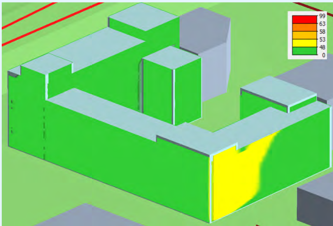
figuur 6: geluidsbelasting als gevolg van de Overschiestraat (inclusief aftrek) (zuidwest aanzicht)
