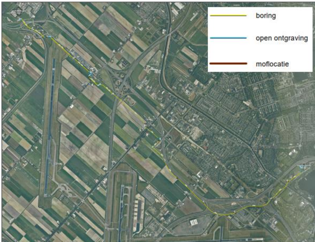
Figuur 1.1 Ligging van het kabeltracé Vijfhuizen - Nieuwe Meer
