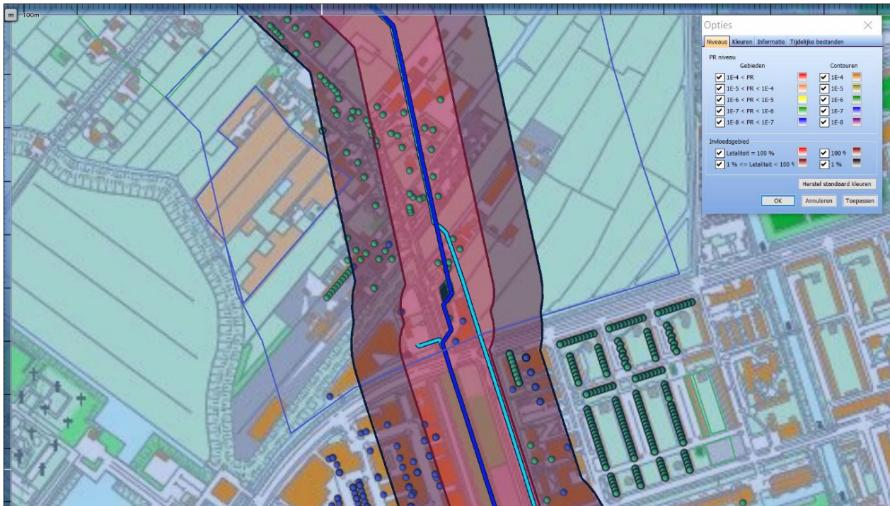
Figuur 7: Invloedsgebied en 100% letaliteitszone leiding 5277_leiding-W-534-24-deel-1.
