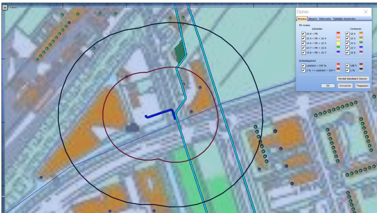
Figuur 8: Invloedsgebied en 100% letaliteitszone leiding 5277_leiding-A-561-deel-1 .
