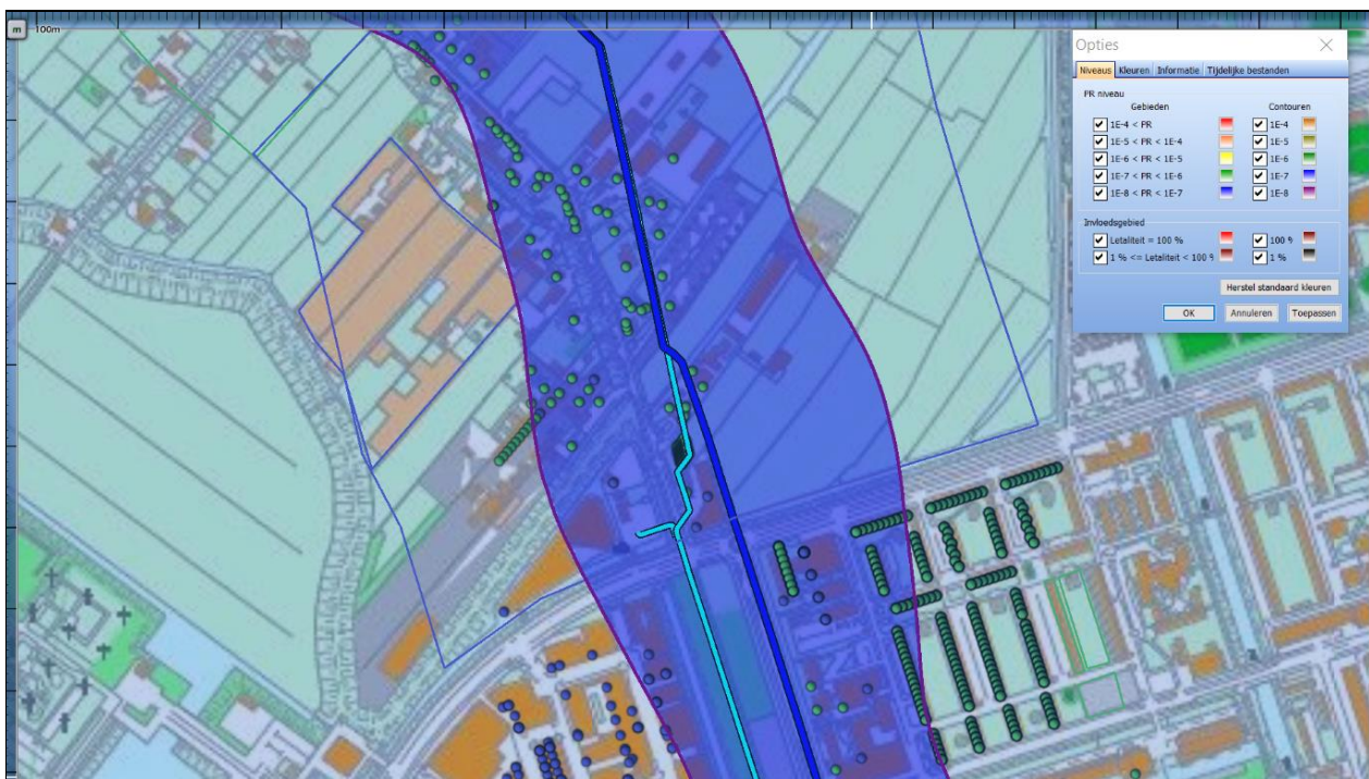
Figuur 4: Plaatsgebonden risicocontouren leiding 5277_leiding-A-561-deel-1 .
