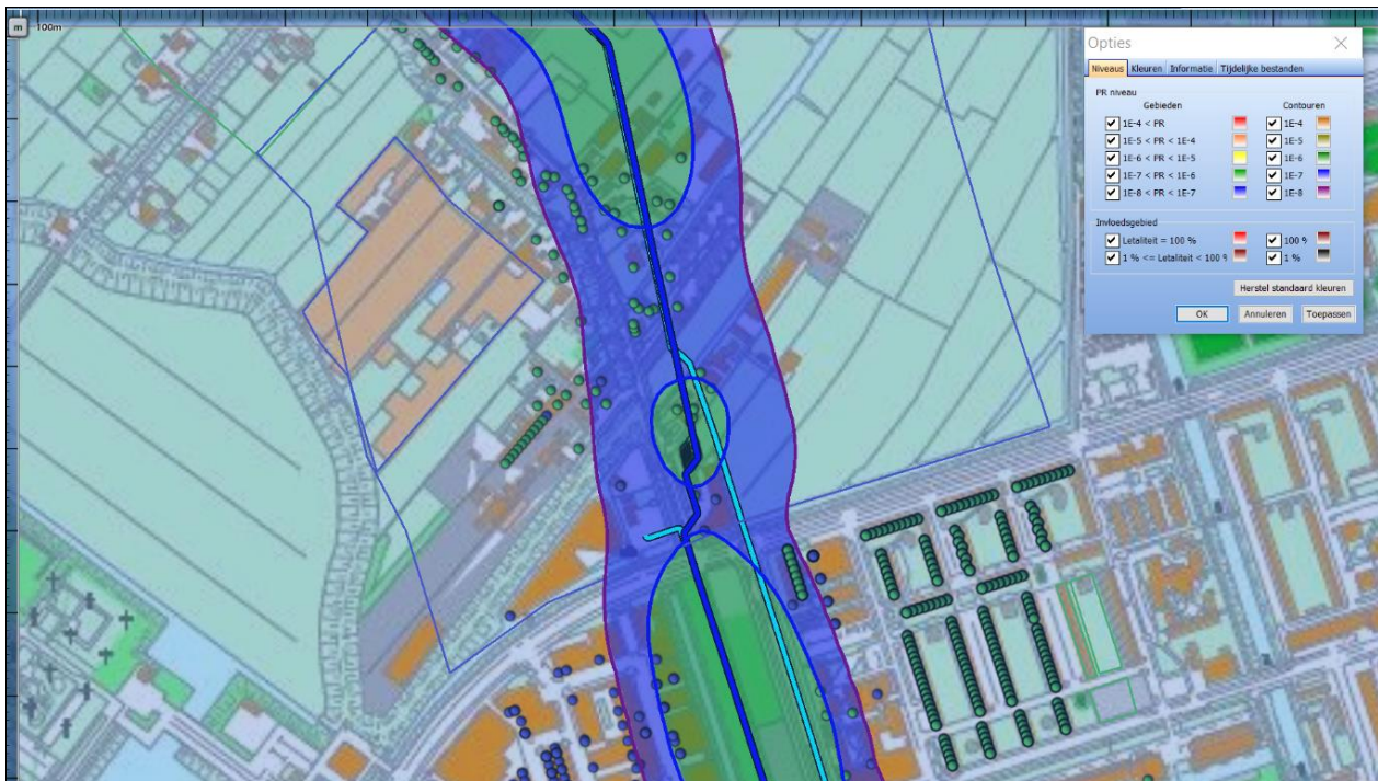
Figuur 3: Plaatsgebonden risicocontouren leiding 5277_leiding-W-534-01-deel-1.
