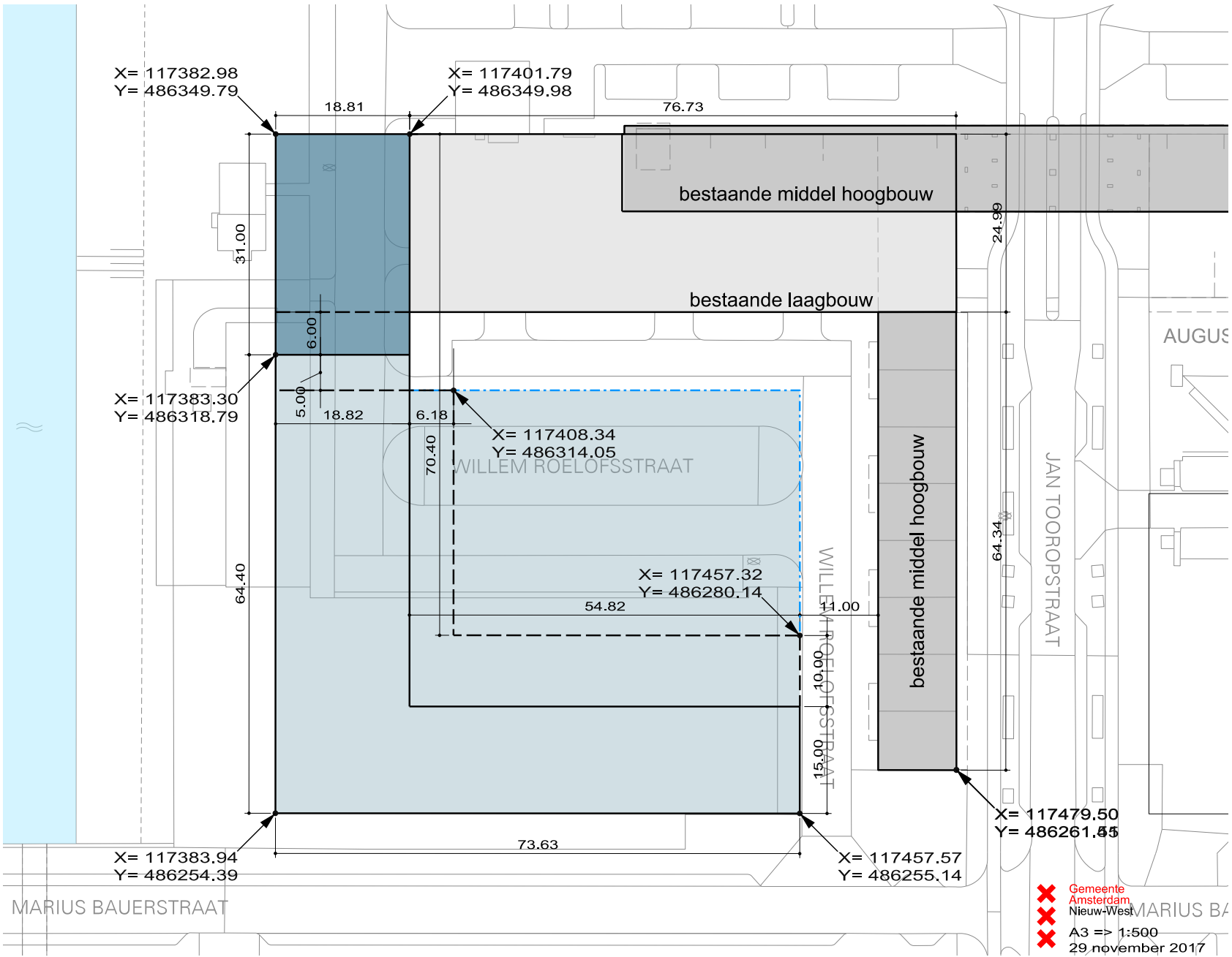
Afmetingen Blok 6
