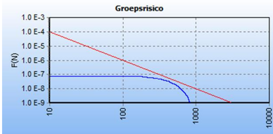
Figuur 9: Groepsrisicocurve behorend bij leidingdeel met het hoogste groepsrisico (leiding 751-leiding-A-561-deel-1).
