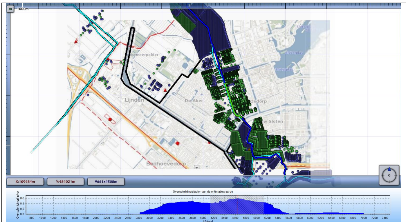
Figuur 8: Verloop van het groepsrisico (751-leiding-A-561-deel-1) als fractie van de oriëntatiewaarde van het groepsrisico. Het gearceerde gebied geeft het groepsrisico van het groen gekleurde stuk leiding aan.
