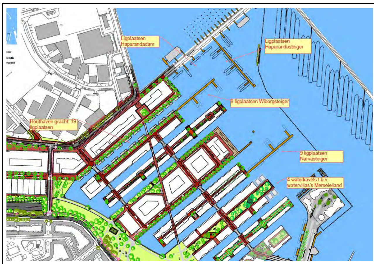
Figuur 1.1: Situatie projectlocatie met nieuwe ligplaatsen en steigers
