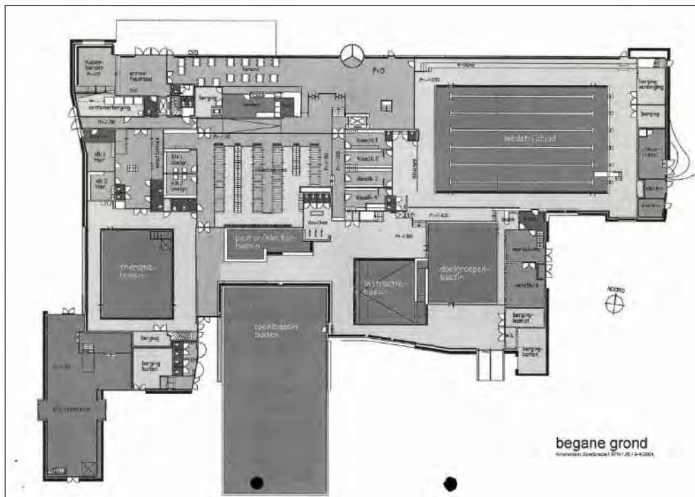
Figuur 8.2 Plattegrond begane grond Sportplaza Mercator
