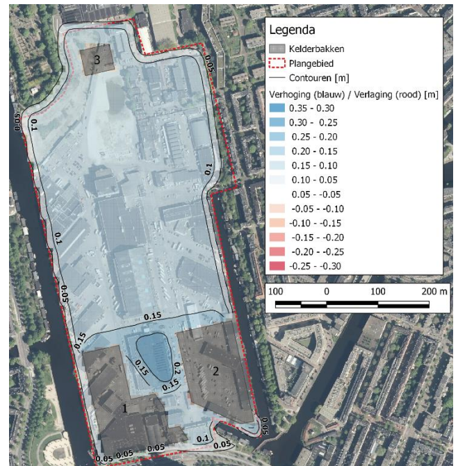
Figuur 15. Effect verhoging grondwaterstand t.o.v. gemiddelde waterstand situatie na 10 dagen (bui T2) en 80mm neerslag, inclusief effect kelders en 50% extra infiltratie t.o.v. huidige situatie en 100% toename infiltratie ter plaatse van de Marktweide.
