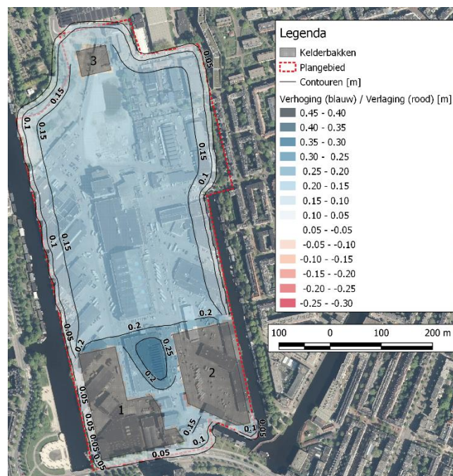
Figuur 21. Grondwaterstand verhoging tussen toekomstige W_h2050 situatie en de situatie W_h2050 met bui T2 na 10 dagen.
