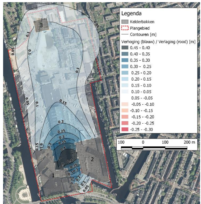
Figuur 19. Grondwaterstand verhoging tussen huidige GG situatie en de toekomstige Wh 2050 situatie. Inclusief kelders en toename onverhard oppervlak.
