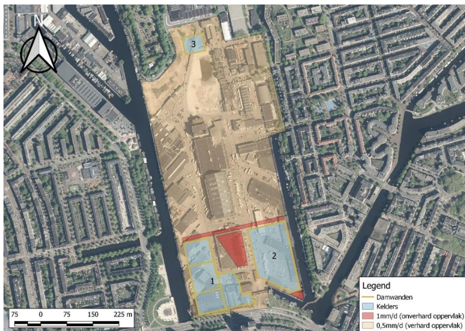
Figuur 10. Toekomstige situatie locatie kelders en damwand en verhard/onverhard oppervlak.
