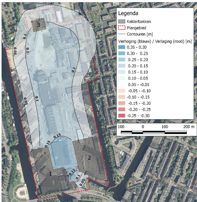
Figuur 18. Grondwaterstand verhoging tussen huidige GG situatie en de toekomstige Wh 2050 situatie. Inclusief kelders, exclusief wijziging onverhard oppervlak. Tussen de kelders wordt een verhoging van maximaal 18 cm berekend.
