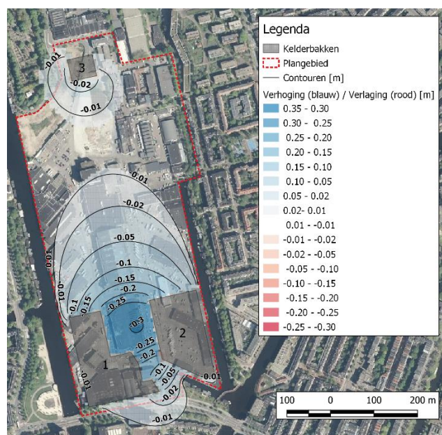
Figuur 12. Effect kelders en wijziging in toename onverhard oppervlak (stationaire) in de huidige gemiddelde grondwater situatie. Verhoging tussen 5 en 30 cm. Let op: verschil in legenda (kleurschaal).
