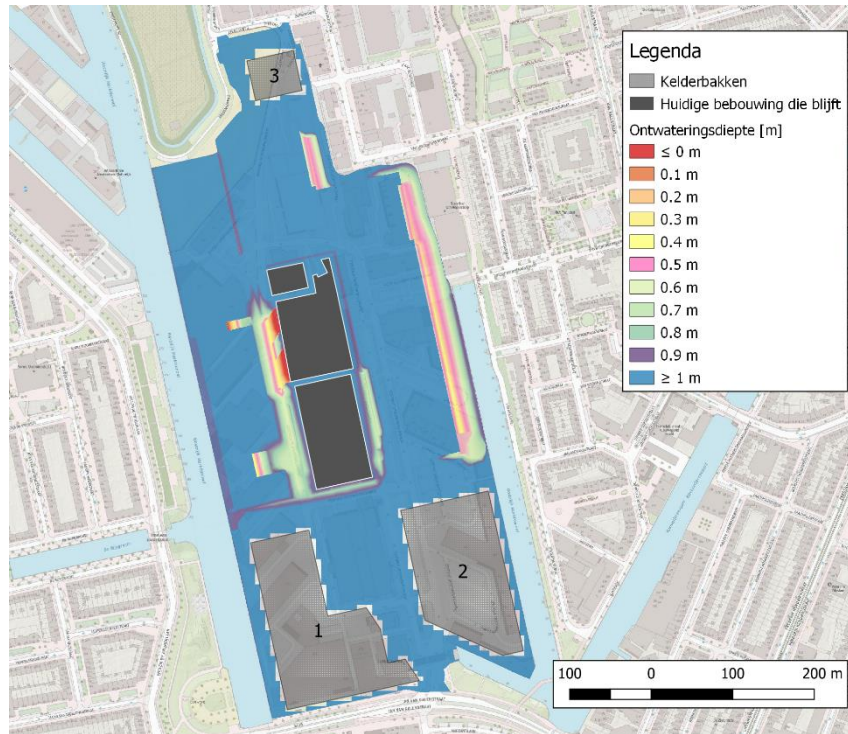
Figuur 26. Ontwateringsdiepte toekomstige situatie (stationair) met kelders en toename onverhard oppervlak. Ter plaatse van de roze locaties wordt 50 cm ontwateringsdiepte berekend. De rode locaties zijn huidige laaddocks.
