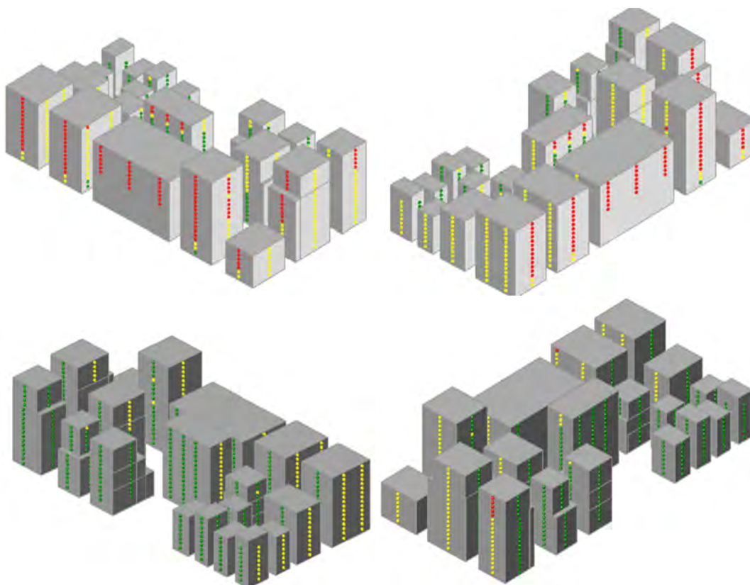
Figuur 4-11 Geluidbelasting per gevelhoogte door industrielawaai. (groen L_{den} \leq 50 dB; geel 50 \text{ dB} < L_{den} \leq 55 dB; rood L_{den} > 55 dB).
