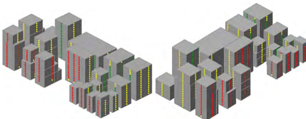
Figuur 4-6 Geluidbelasting per gevelhoogte door spoorwegen zonder maatregelen. (groen L_{den} \leq 55 dB; geel 55\text{dB} < L_{den} \leq 65\text{dB} ; rood L_{den} > 65\text{dB} )
