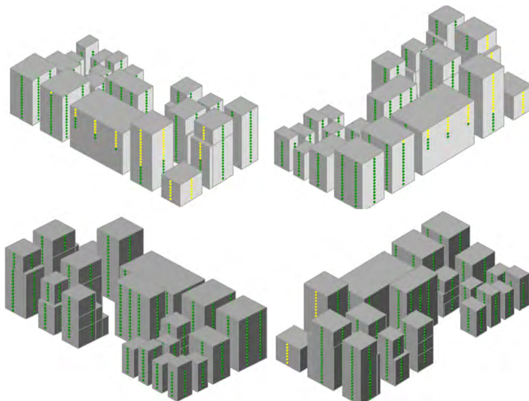
Figuur 4-4 Geluidbelasting per gevelhoogte door lokale wegen. (groen L_{den} \leq 53 dB; geel 53\text{dB} < L_{den} \leq 70\text{dB} ; rood L_{den} > 70 dB).
