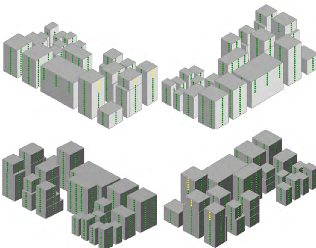
Figuur 4-2 Geluidbelasting per bouwlaag door rijkswegen. (groen L_{den} \leq 50 dB; geel 50\text{dB} < L_{den} \leq 60\text{dB} ; rood L_{den} > 60\text{dB} ).
