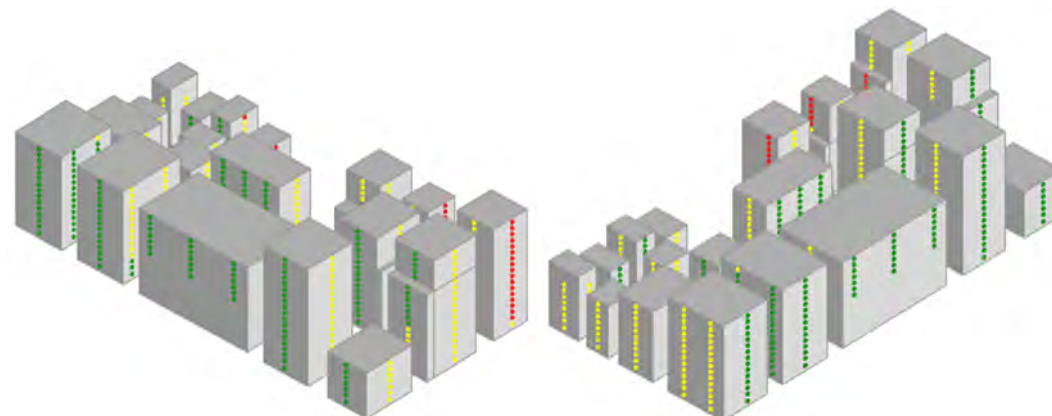
Figuur 4-5 Overschrijding van de standaardwaarde (geel) en van de grenswaarde (rood) per gevel.
