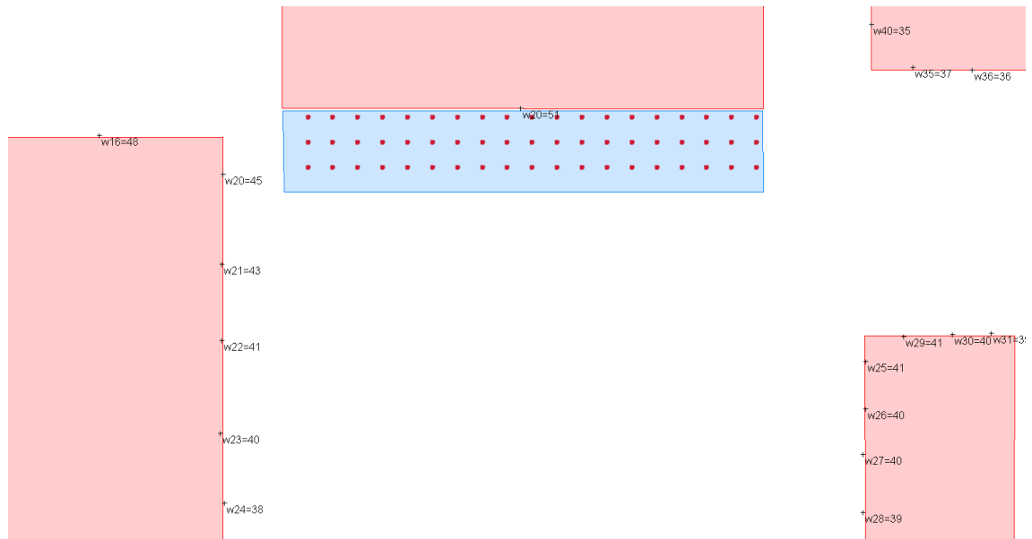
Figuur 4-10 maximale geluidbelasting in de nachtsituatie met 100 personen op het terras, waarvan 50% tegelijkertijd spreekt.
