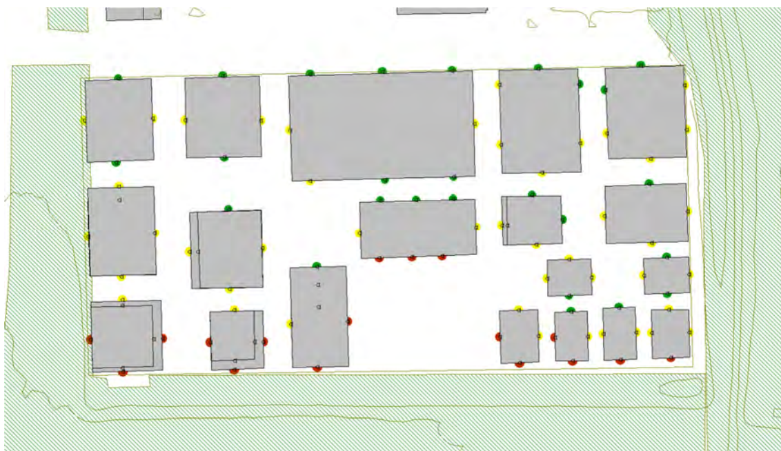
Figuur 4-5 Overschrijding van de standaardwaarde (geel) en van de grenswaarde (rood) per gevel.
