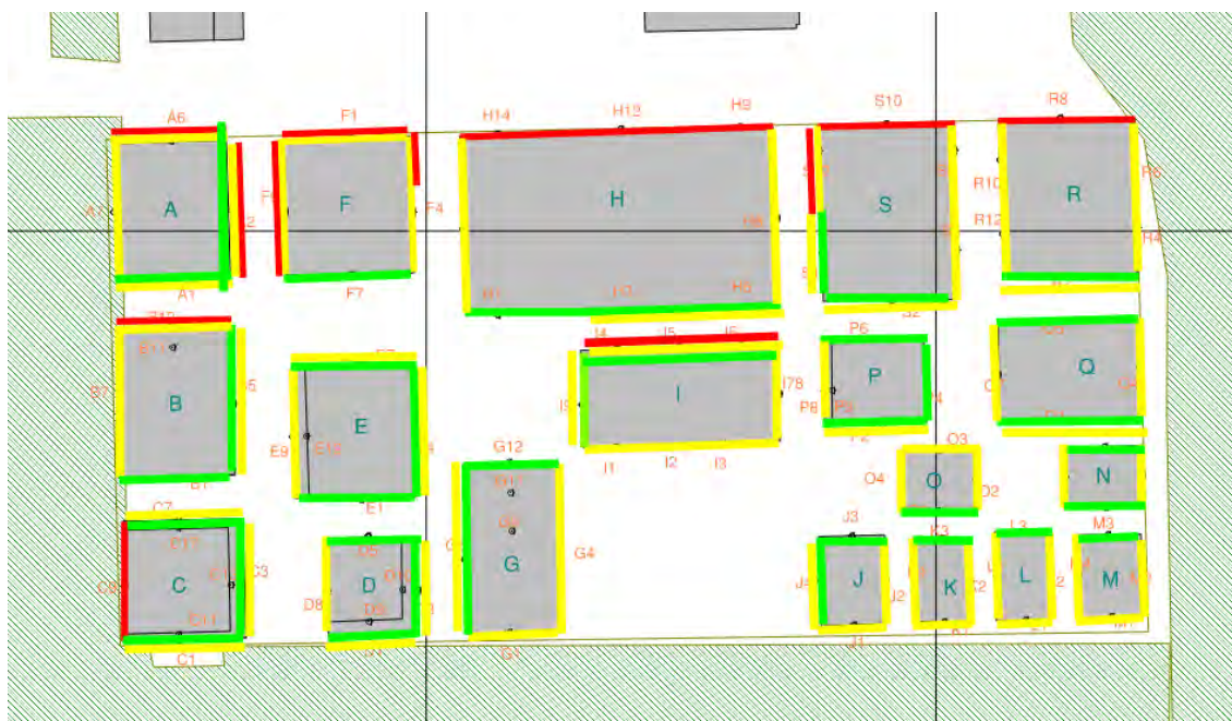
Figuur 7-1 Overzicht gevels geluidluw (groen), overschrijding standaardwaarde/voorkeursgrenswaarde (geel) en overschrijding grenswaarde/maximale ontheffingswaarde (rood).
