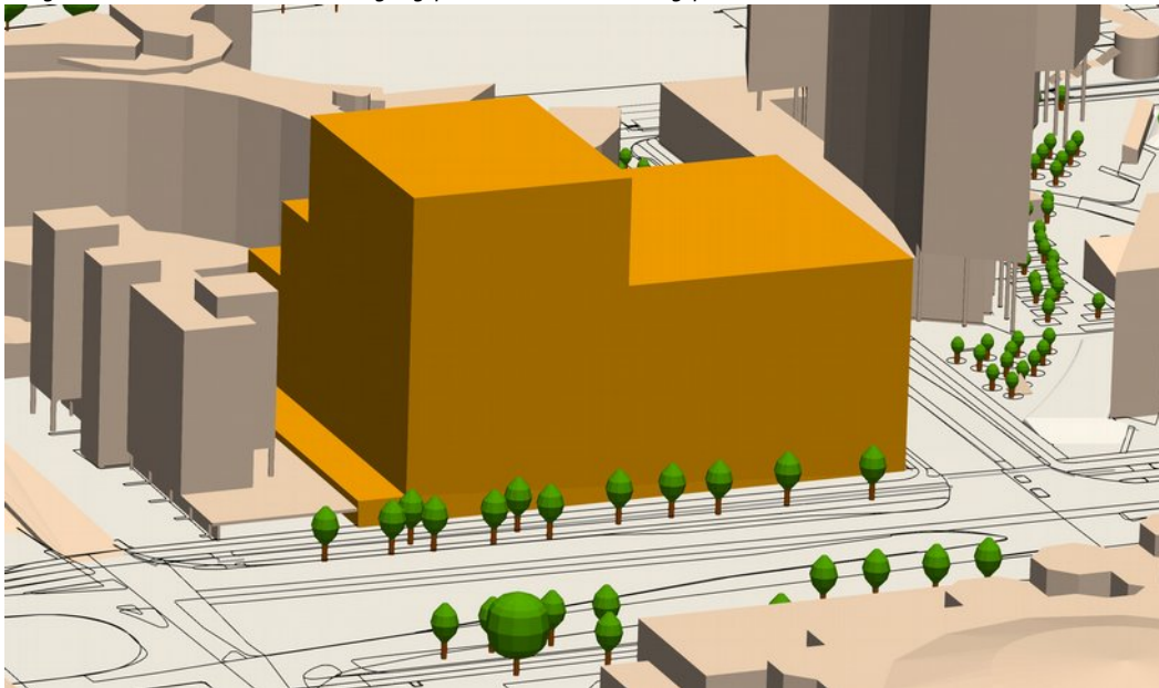
f1.3 Het gehanteerde 3D-model van het uitgangspunt van het bestemmingsplan
