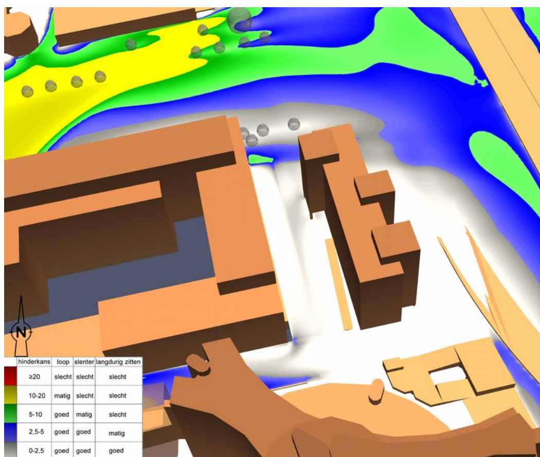
f3.7 Het te verwachten windklimaat op de terrassen naar de maatvoering van het geplande ontwerp, beoordeeld volgens NEN 8100 (beoordelingsvlak 1,75 m boven terrasniveau)
