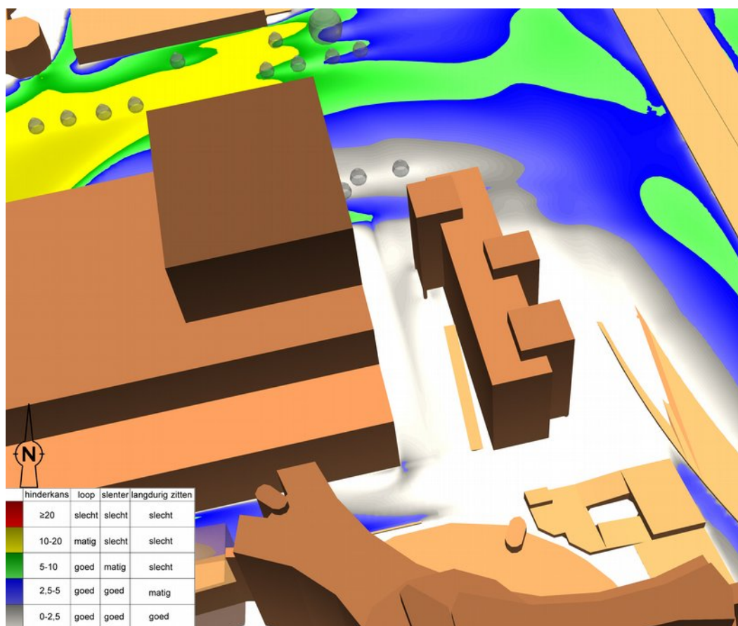
f3.8 Het te verwachten windklimaat op de terrassen naar de maatvoering van het bestemmingsplan, beoordeeld volgens NEN 8100 (beoordelingsvlak 1,75 m boven terrasniveau)
