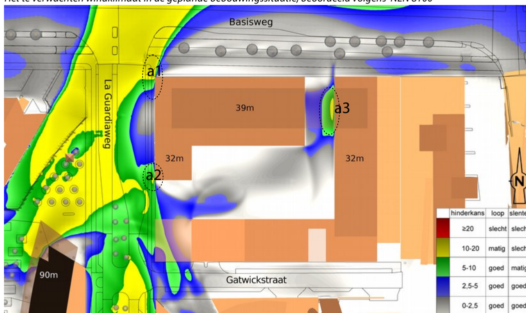
f3.4 Het te verwachten windklimaat in de geplande bebouwingssituatie, beoordeeld volgens NEN 8100
