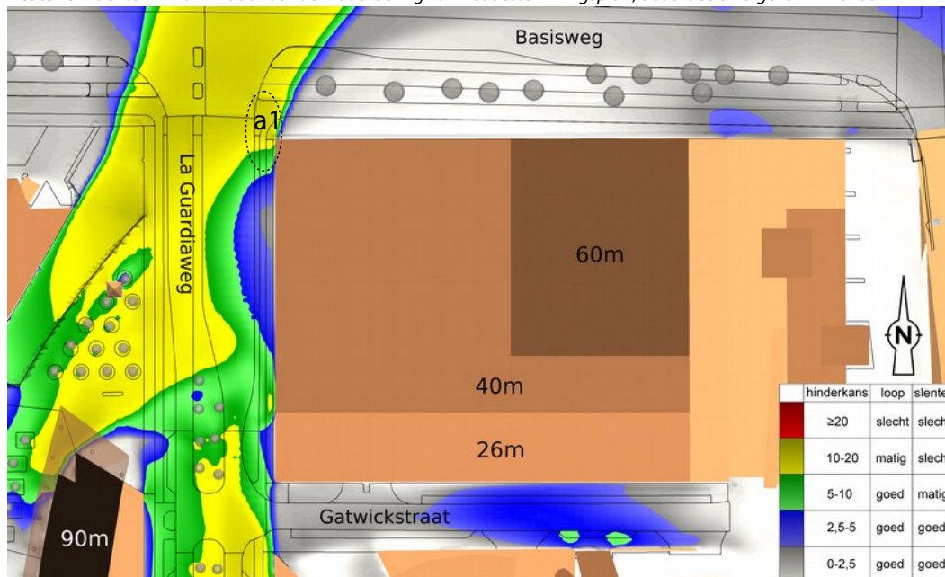
f3.6 Het te verwachten windklimaat naar de maatvoering van het bestemmingsplan, beoordeeld volgens NEN 8100
