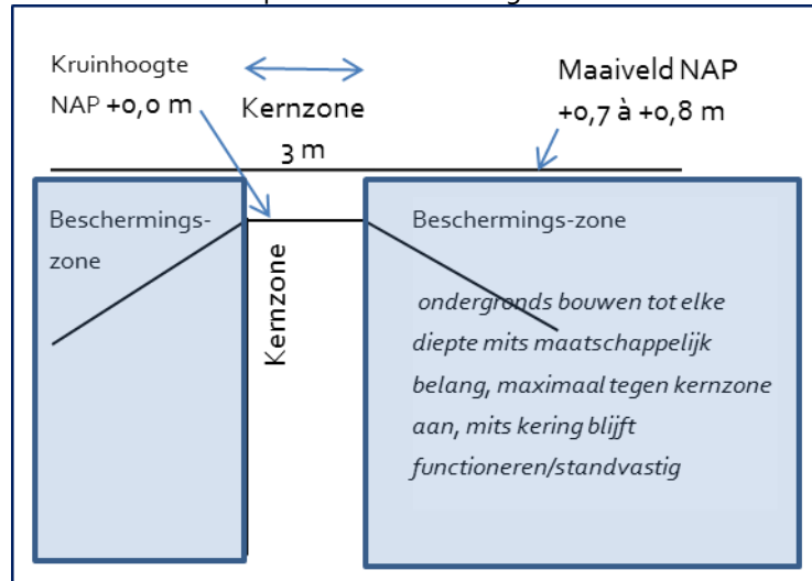
Figuur 16 principe van ondergronds bouwen in de beschermingszones van een verholen kering
