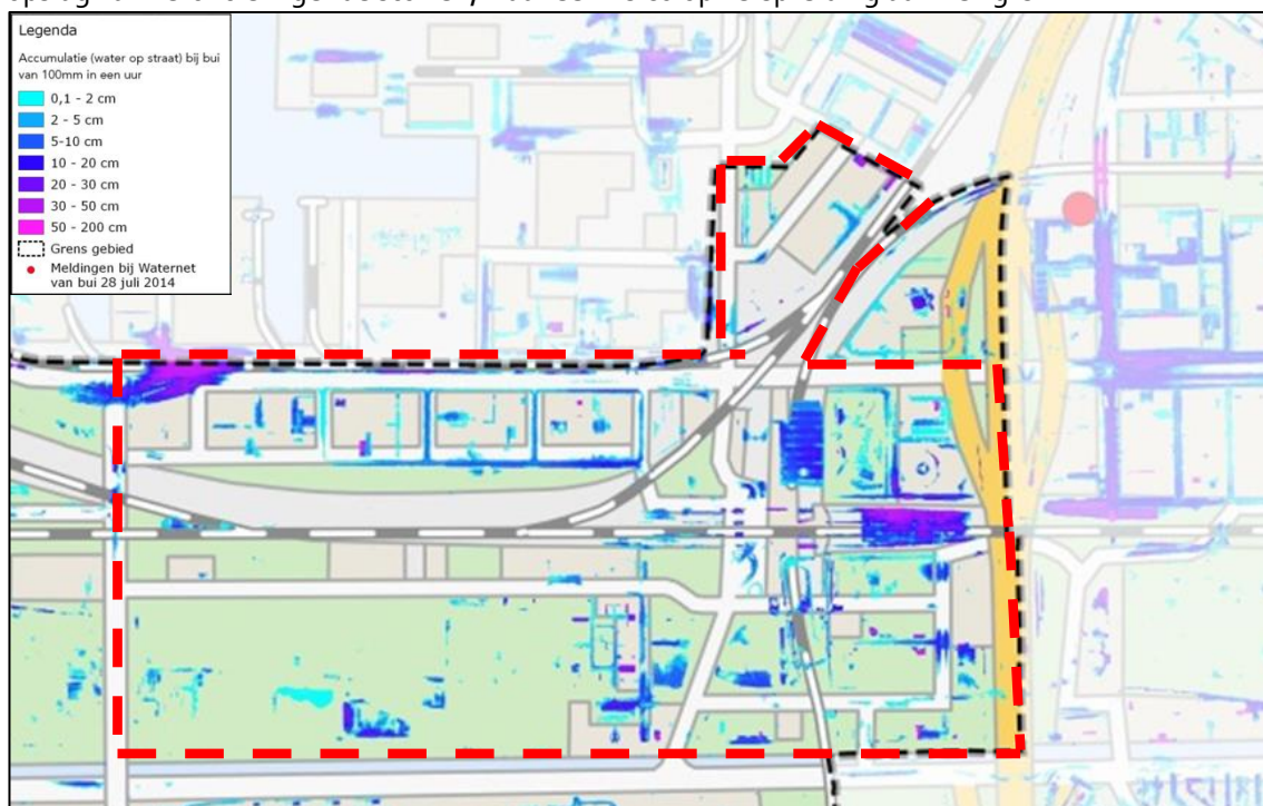
Figuur 7: Simulatie water op straat (WOLK) bij 100 mm neerslag in een uur (Bron 4), met indicatie van plangebied Sloterdijk-Centrum/II inclusief sporen binnen rode stippellijnen
