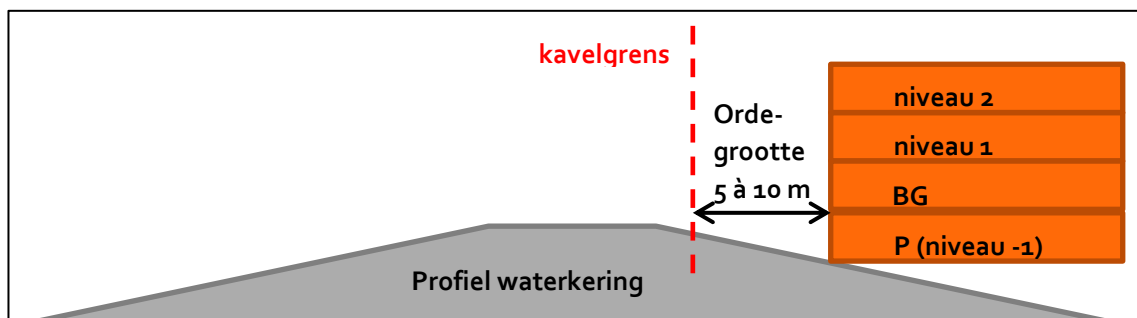
Figuur 13 Principe van een éénlaags parkeergarage nabij de waterkering; in de laatste 5 à 10 m van de kavel kan de kelder niet op diepte worden gerealiseerd omdat die buiten het waterkeringsprofiel moet blijven; maten zijn per locatie verschillend.
