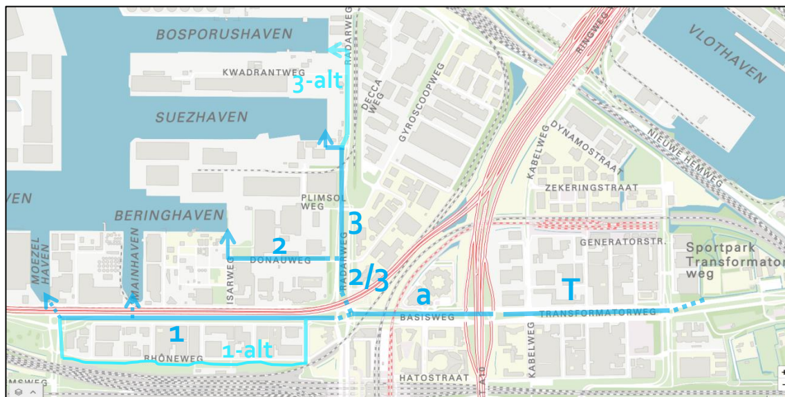
Figuur 11 Varianten voor toekomstige hoofdwatgang
