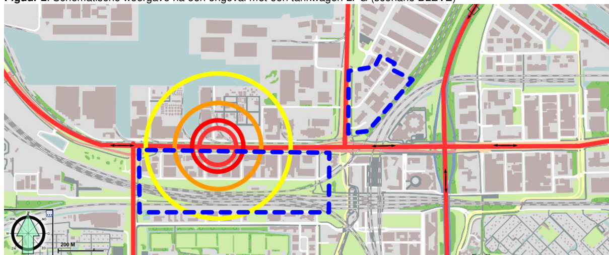
Figuur 2. Schematische weergave na een ongeval met een tankwagen LPG (scenario BLEVE)
