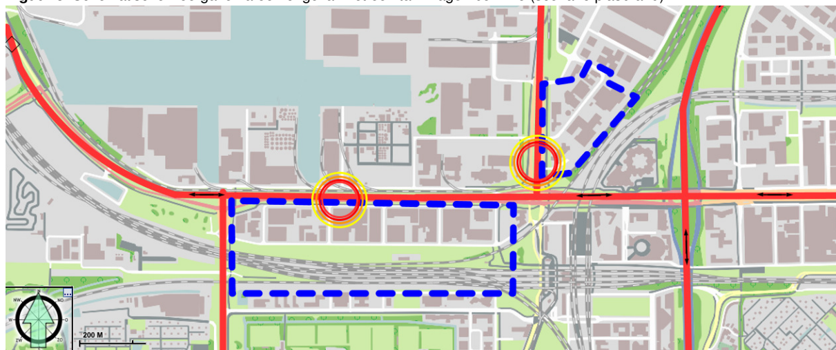
Figuur 3. Schematische weergave na een ongeval met een tankwagen benzine (scenario plasbrand).
