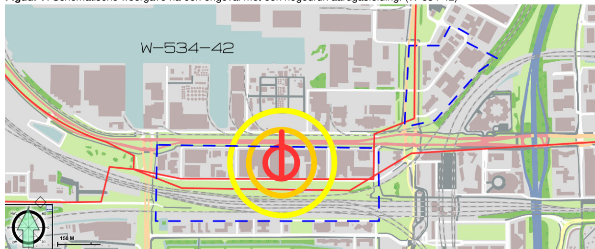
Figuur 7. Schematische weergave na een ongeval met een hogedruk aardgasleiding. (W-534-42)
