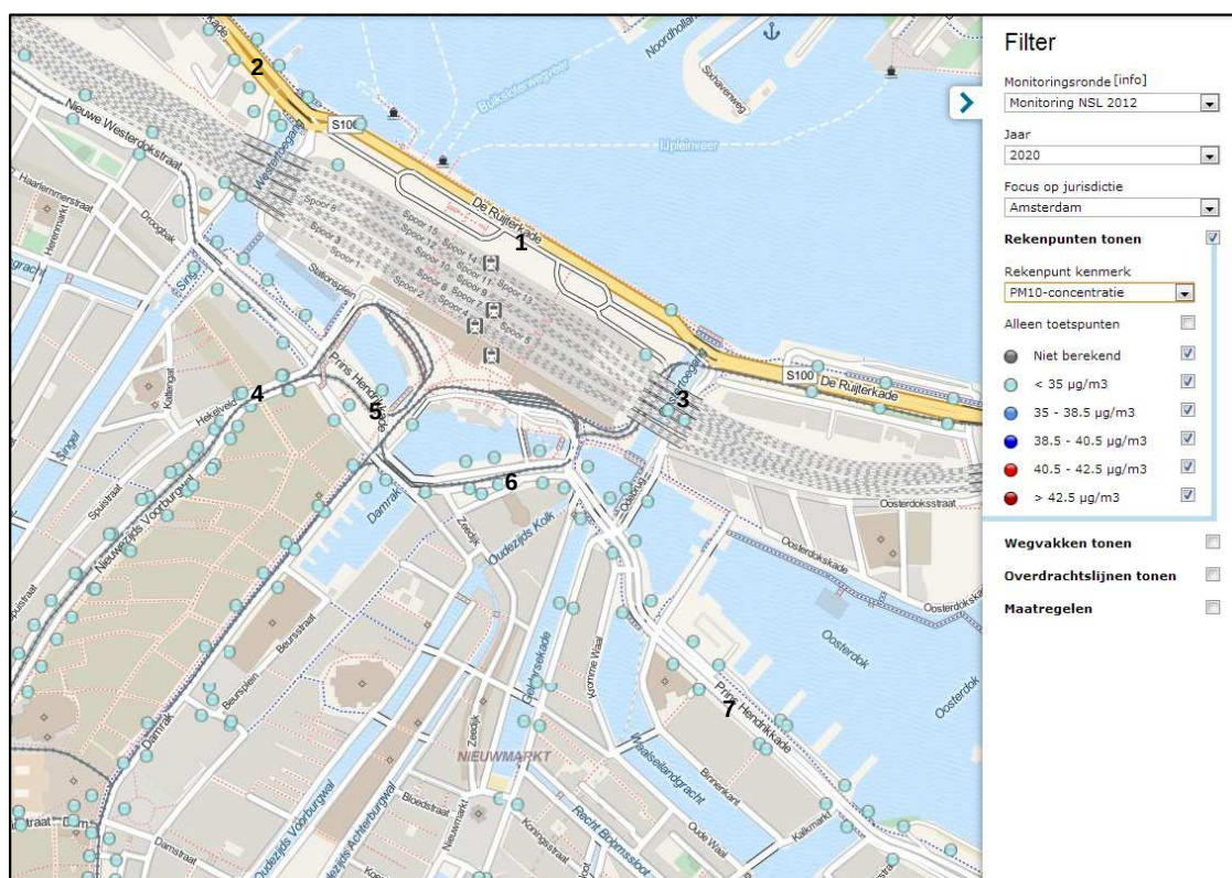
figuur 7 concentraties PM 10 in 2023 (NSL monitoringsjaar 2020)
