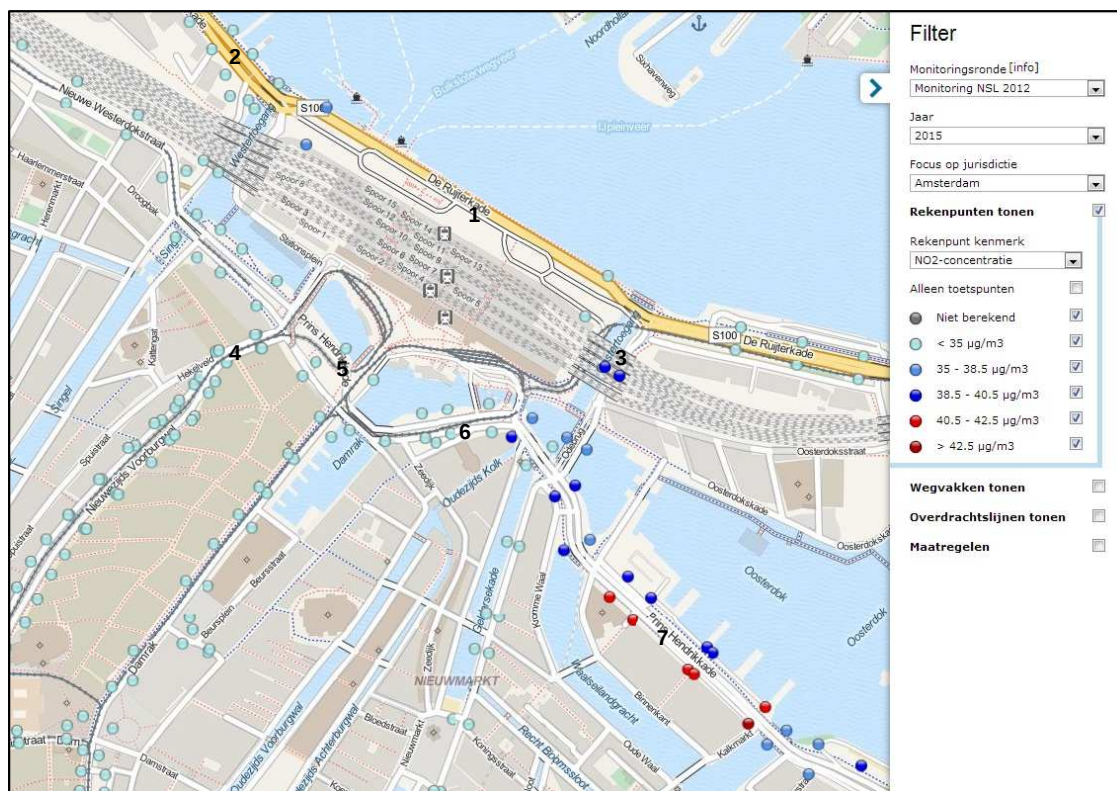
figuur 4 concentraties NO 2 in 2015
