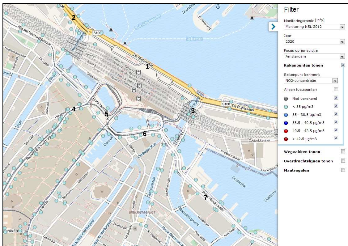
figuur 6 concentraties NO 2 in 2023 (NSL monitoringsjaar 2020)
