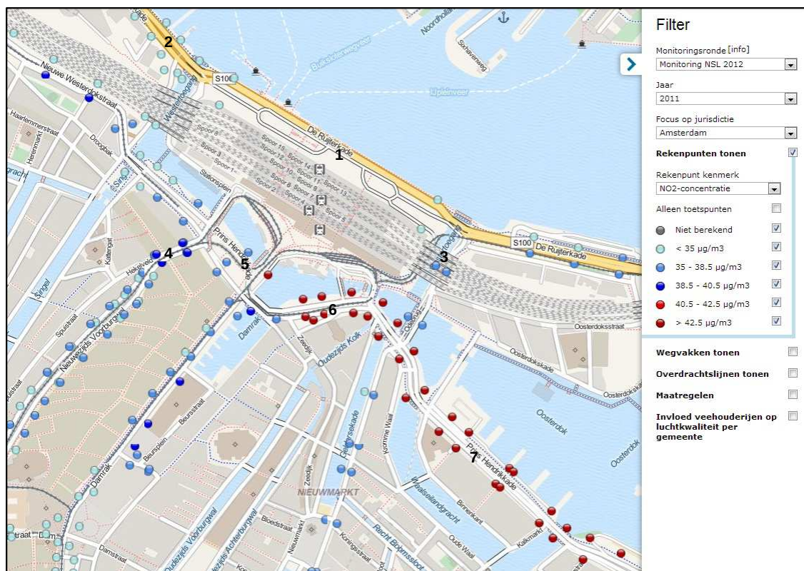
figuur 2 concentraties NO 2 in 2011
