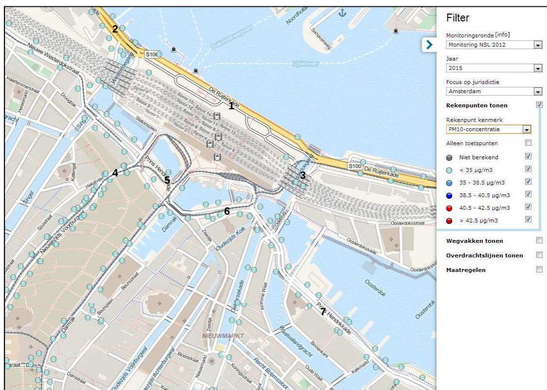
figuur 5 concentraties PM 10 in 2015
