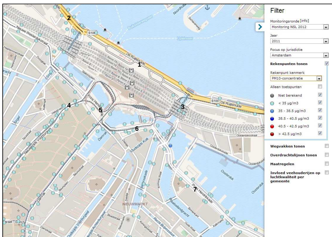
figuur 3 concentraties PM 10 in 2011
