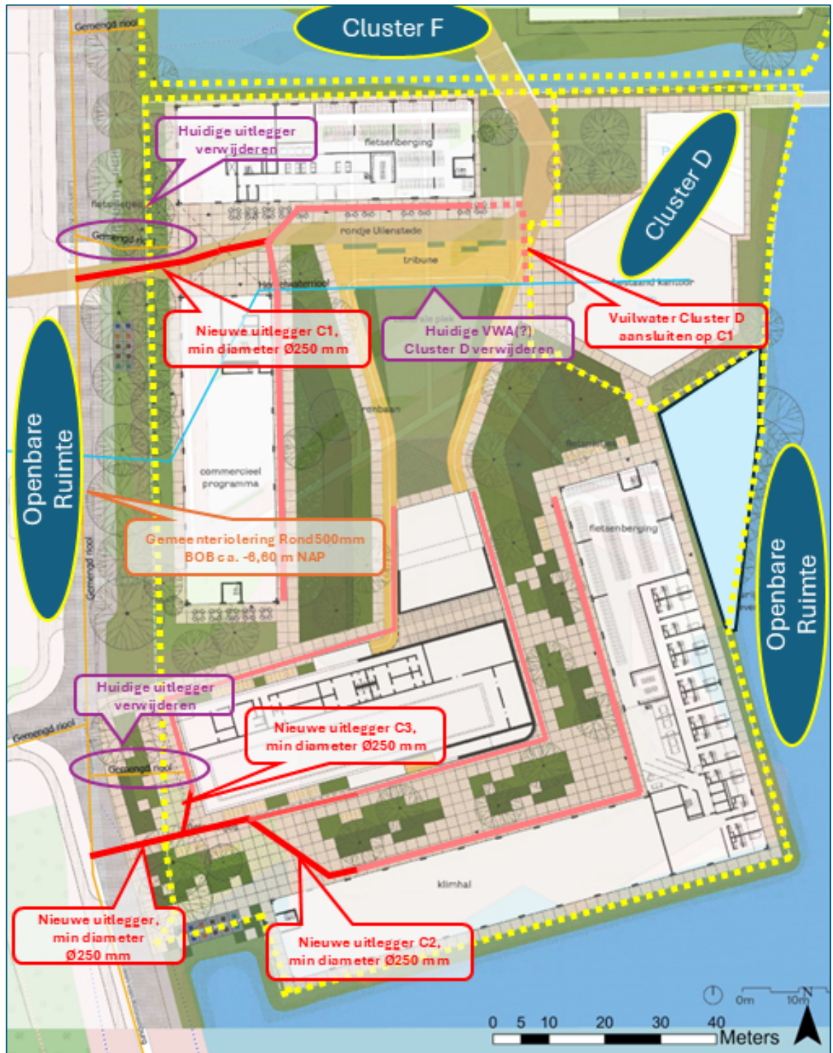
Figuur 4-3 Vuilwaterafvoer met nieuwe aansluitleidingen incl. diameters. Aan te passen naar locatie aankoppelpunt vanuit de panden naar buiten o.b.v. verdere ontwikkeling Definitieve Ontwerpen vanuit Overdevest.
