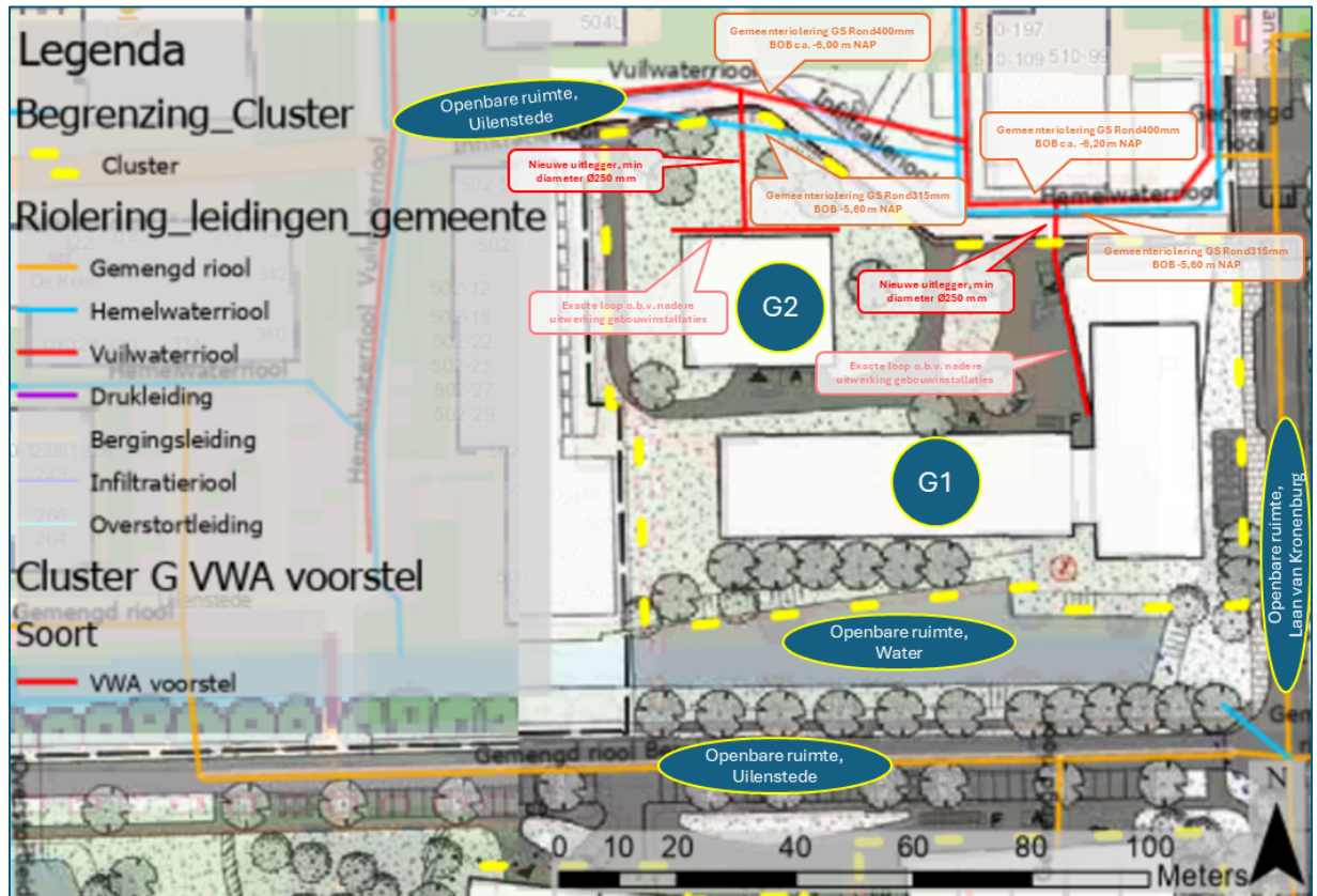
Figuur 7-3 Vuilwaterafvoer met nieuwe aansluitleidingen incl. diameters. Aan te passen naar locatie aankoppelpunt vanuit de panden naar buiten o.b.v. verdere installatietechnische uitwerkingen.
