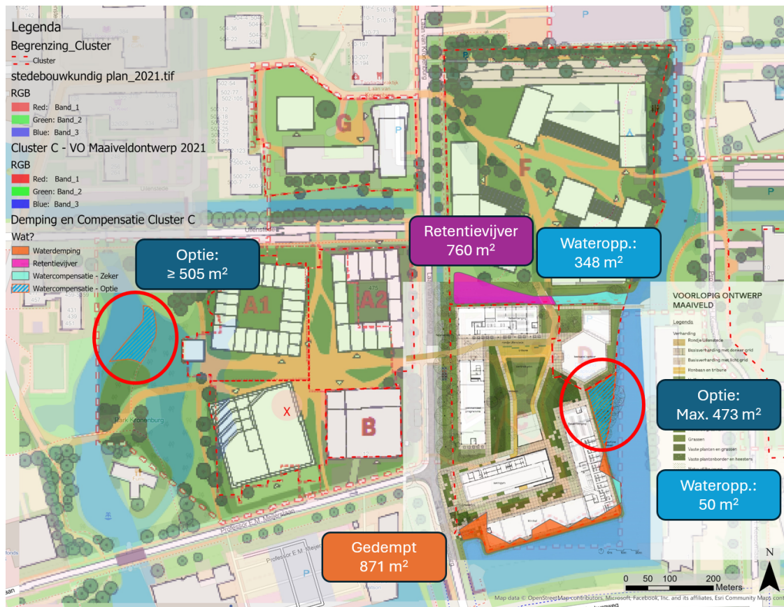
Figuur 4-7 Beschouwing watercompensatie dempen watergangen
