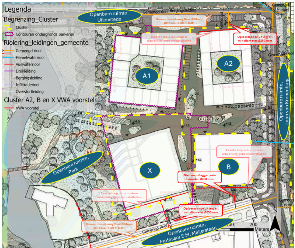
Figuur 6-3 Vuilwaterafvoer met nieuwe aansluitleidingen incl. diameters. Aan te passen naar locatie aankoppelpunt vanuit de panden naar buiten o.b.v. verdere installatietechnische uitwerkingen.
