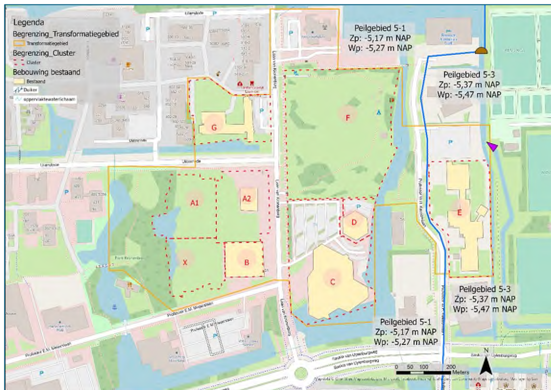
Figuur 2-4 Het huidige watersysteem. Aan oostzijde zit een gemaal en in de noordoosthoek een stuw die zorgt voor 2 peilgebieden.
