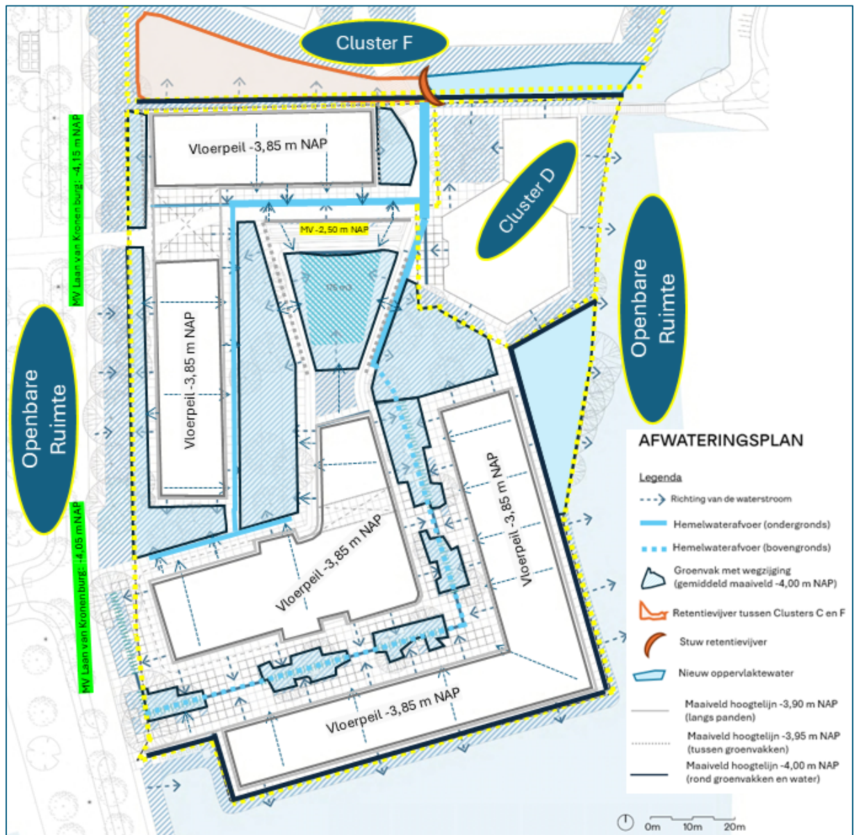
Figuur 4-4 Hemelwaterafvoerstructuur en locatie van waterverwerkende voorzieningen en hoogte-indicatie.
