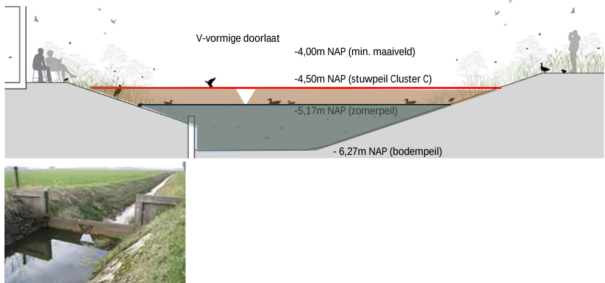
Figuur 4-6 Uitwerking stuw met v-vormige doorlaat retentievijver en impressie.
