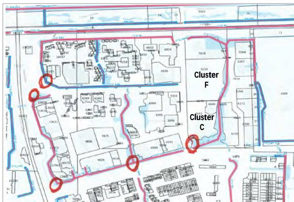
Figuur 5-9: inlaatplaatsen maaiboten onderhoud watersysteem
