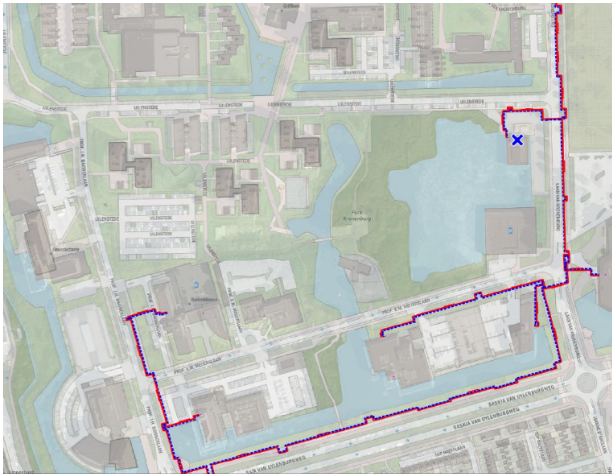
Figuur 2-10 Het warmtenet nabij het Transformatiegebied (2020).
