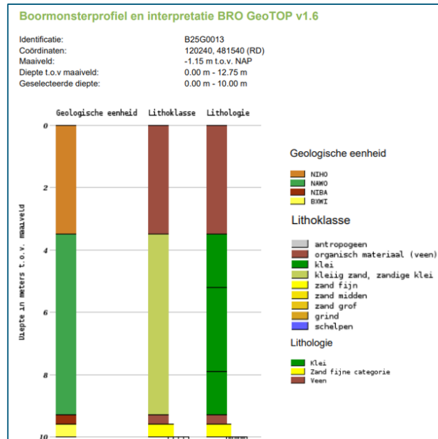
Figuur 2-6 Bodemopbouw nabij Cluster G conform boormonsterprofiel in BRO GeoTOP v1.6.
