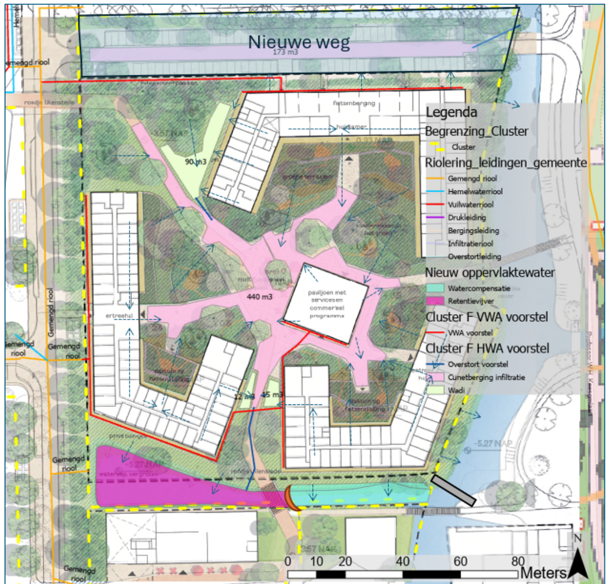
Figuur 5-5: Hemelwaterafvoerstructuur, indicatieve locatie van waterverwerkende voorzieningen en hoogte-indicatie van maaiveld.
