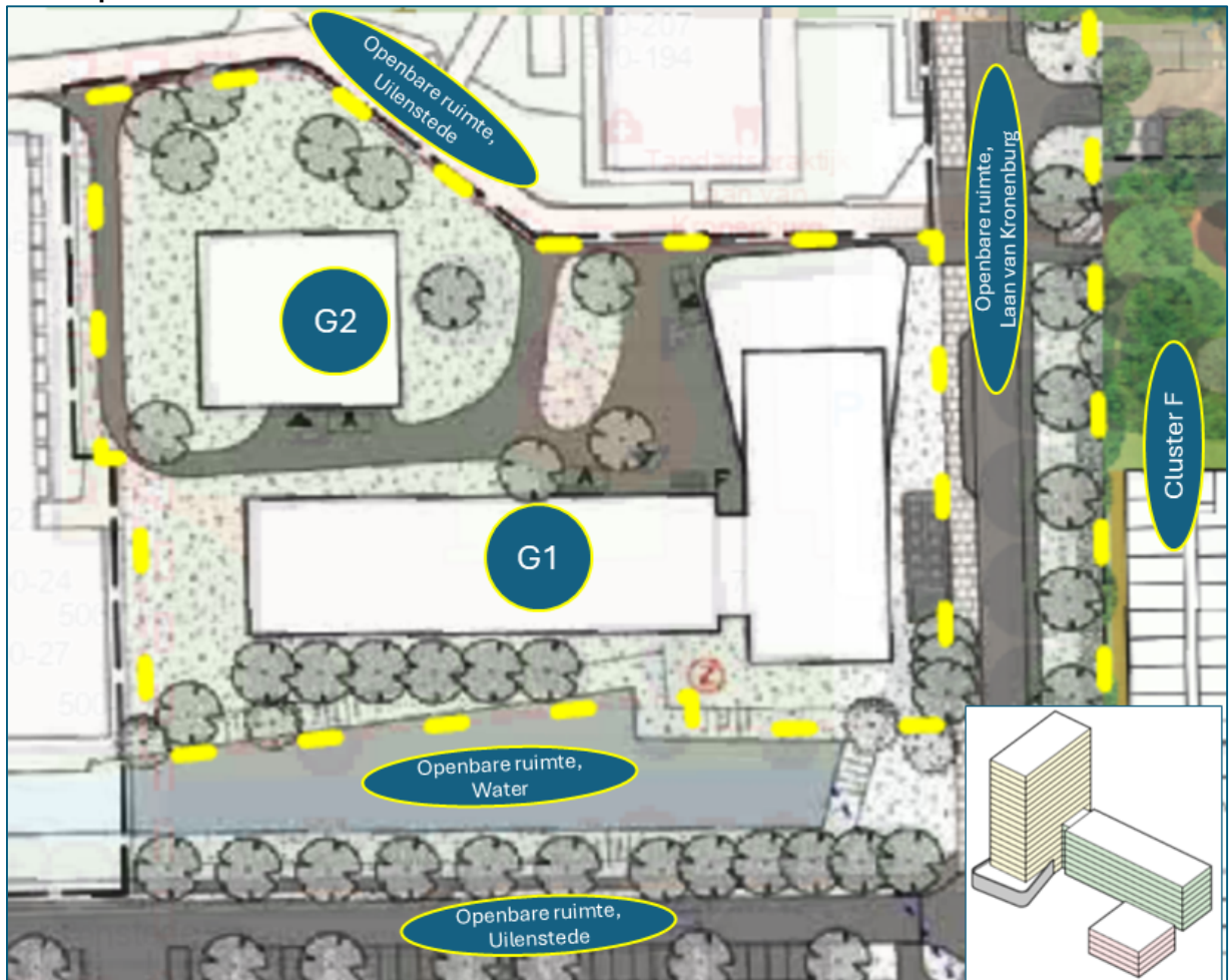
Figuur 7-1: Overzicht van het Cluster G in beoogde situatie, uit VO van BOOM Landscape (2020-09-23). Inzet uit Bouwenvelop.
