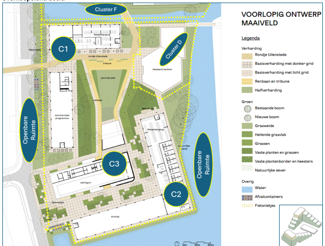
Figuur 4-1 Overzicht van het Cluster C in beoogde situatie, uit Voorlopig Ontwerp LOLA (2021-11-19). Inzet uit Bouwenvelop.
