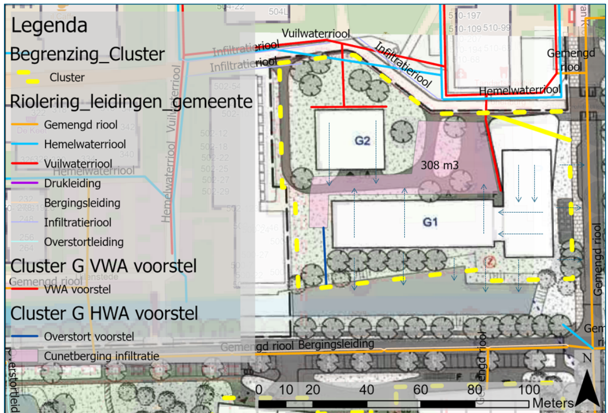
Figuur 7-4 Hemelwaterafvoerstructuur, indicatieve locatie van waterverwerkende voorzieningen.
