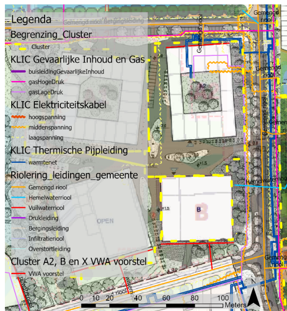
Figuur 6-4 Clusters A2 en B met omliggende ondergrondse infrastructuur uit de KLIC.
