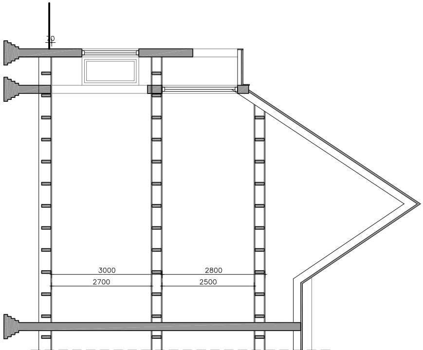
Doorsnede A
