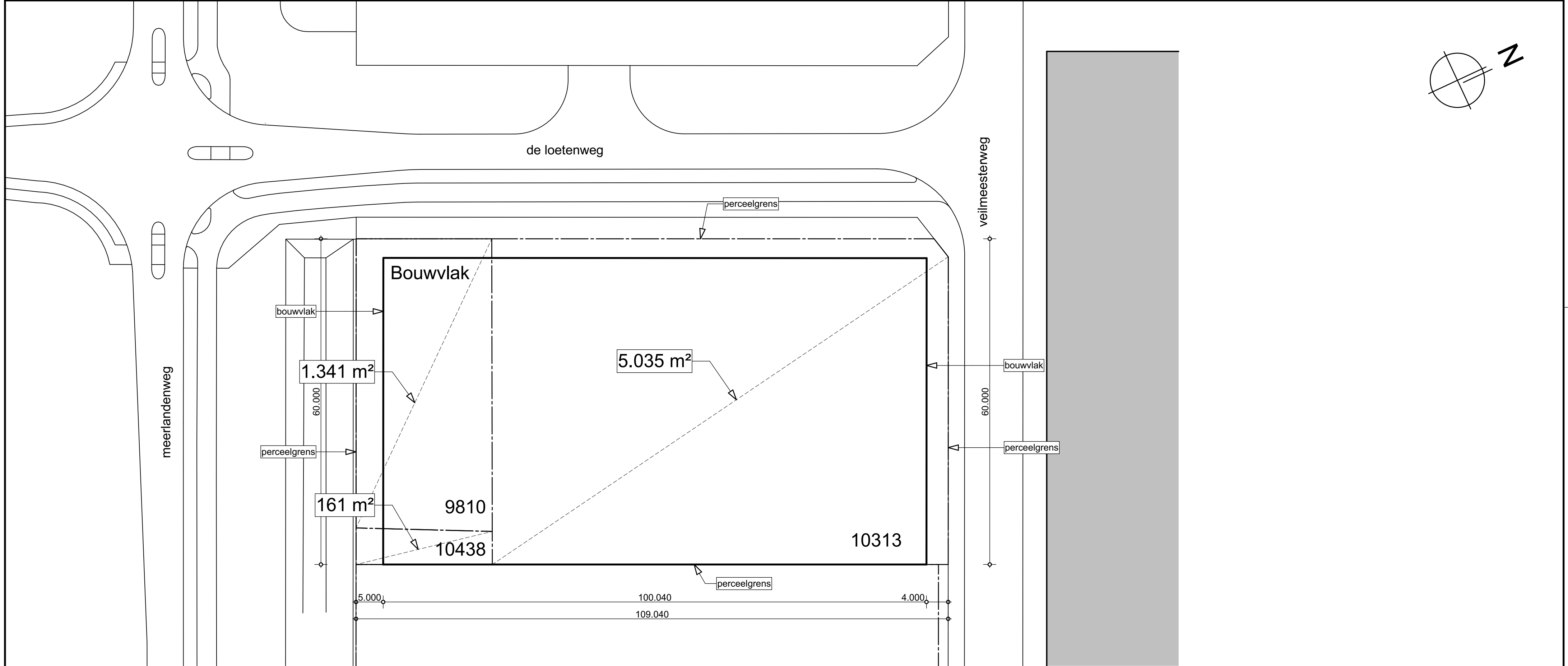
Situatie BESTAAND
