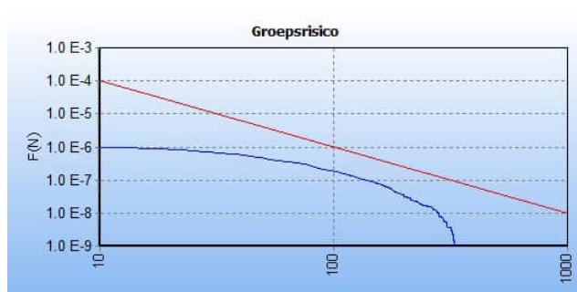
Figuur 7 FN-curve van de kilometer met de hoogste overschrijdingsfactor van gastransportleiding W-540-01 in de huidige situatie. De ligging van deze kilometer is hiernaast in het rood weergegeven op een topografische kaart.
