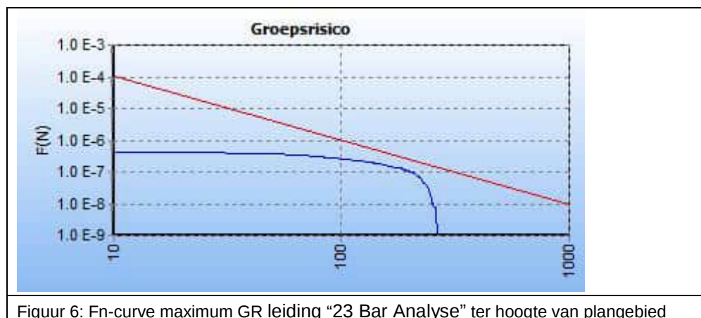
Figuur 6: Fn-curve maximum GR leiding “23 Bar Analyse” ter hoogte van plangebied
