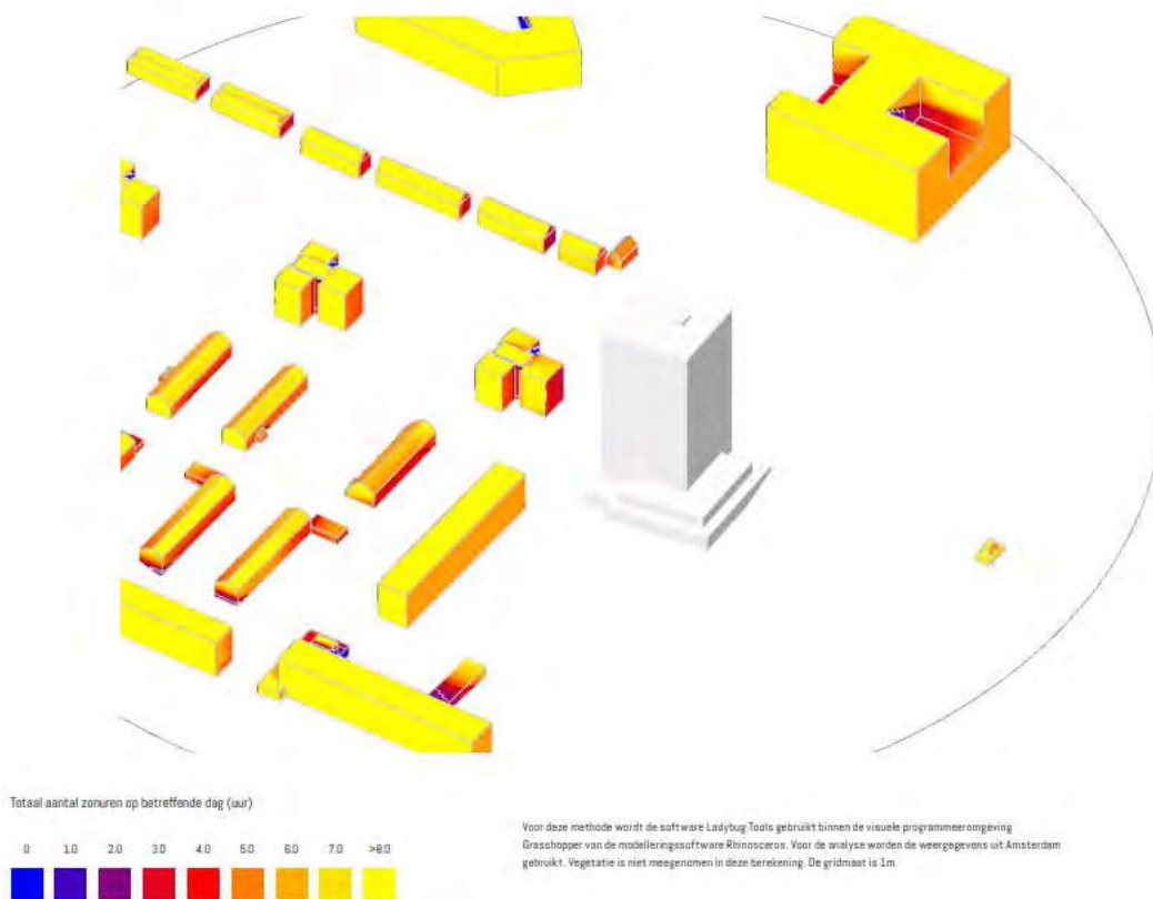
Figuur 4.16 Bezonnning op gevels 19 februari (bron: DGMR)
