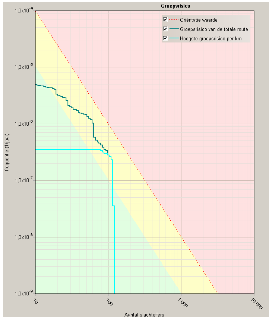
Figuur 5: fN-curve voor groepsrisico in 2020 bij categorie I tunnel
