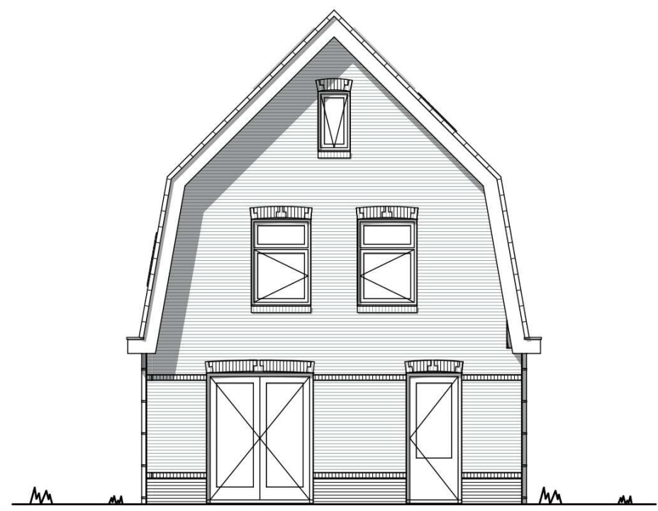
Achtergevel
