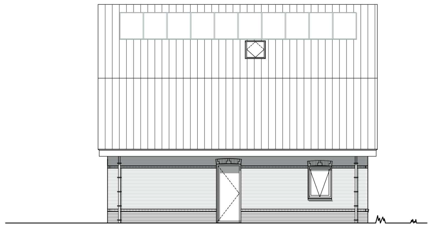
Linkergevel
