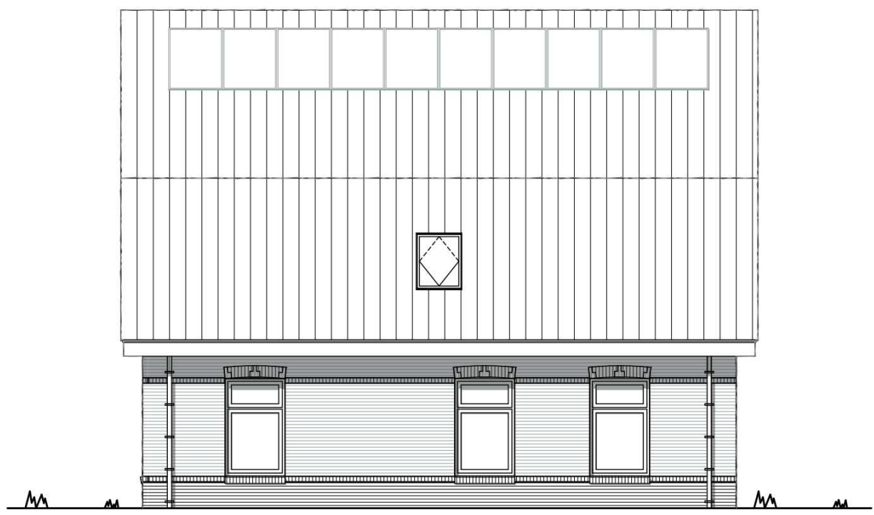
Rechtergevel
