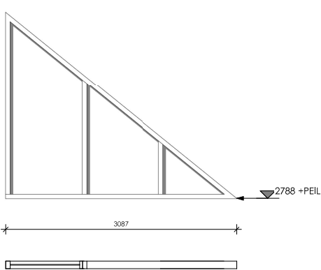
Merk M Pui verdieping achtergevel aantal: 1
