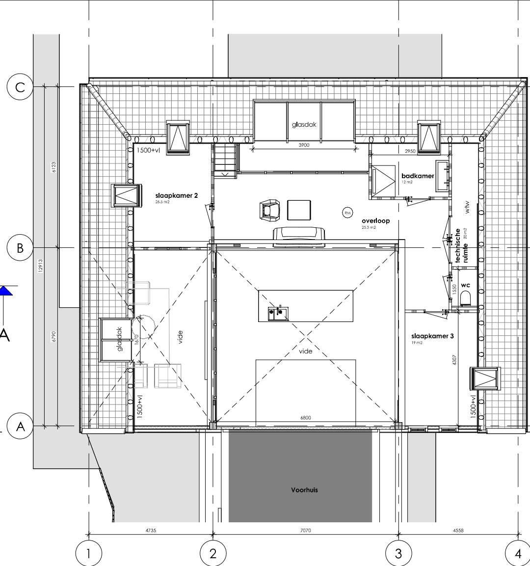
Eerste verdieping
