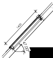
Velux dakraam GGL MK08 Dakraam aantal: 6
