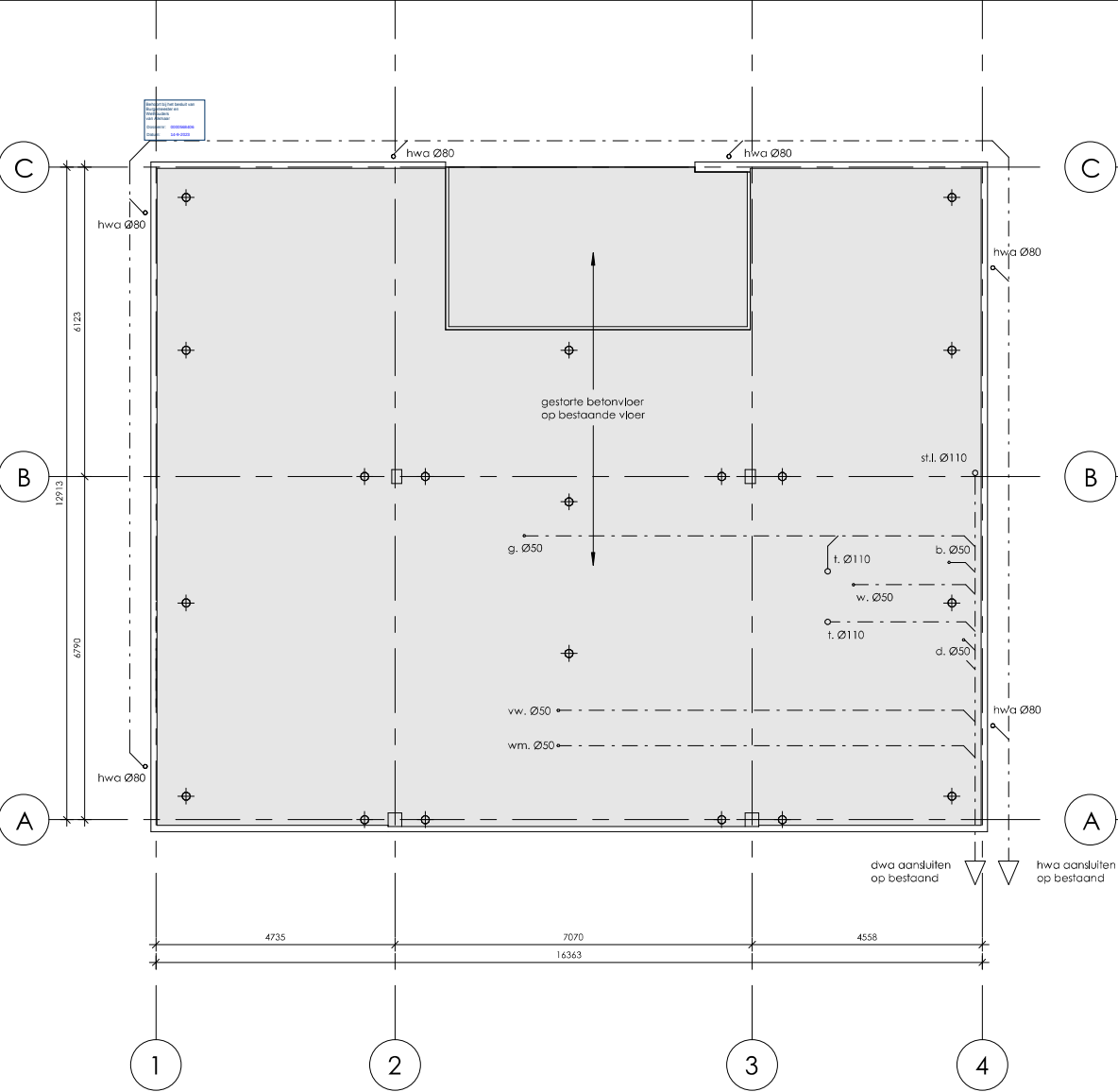
Begane grondvloer bestaande vloer handhaven, betonvloer op bestaande vloer opstorten tot peil
