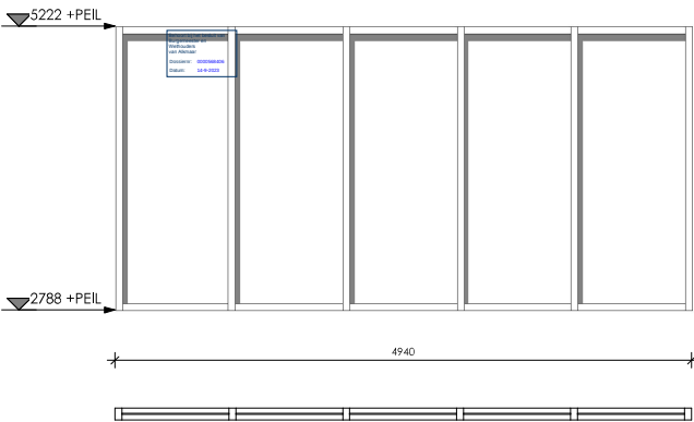
Merk N Pui verdieping achtergevel aantal: 1
