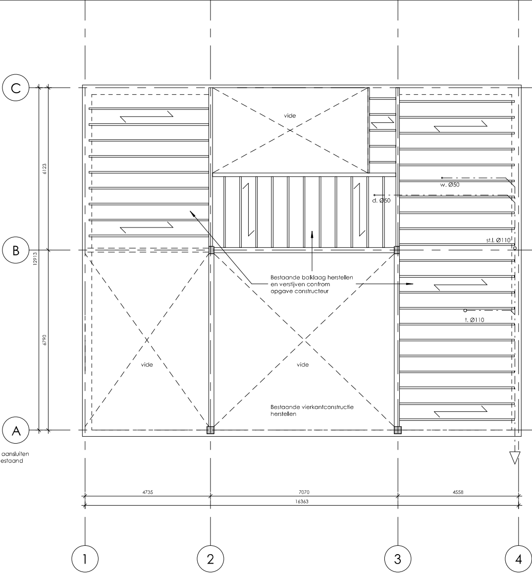
Eerste verdiepingsvloer
