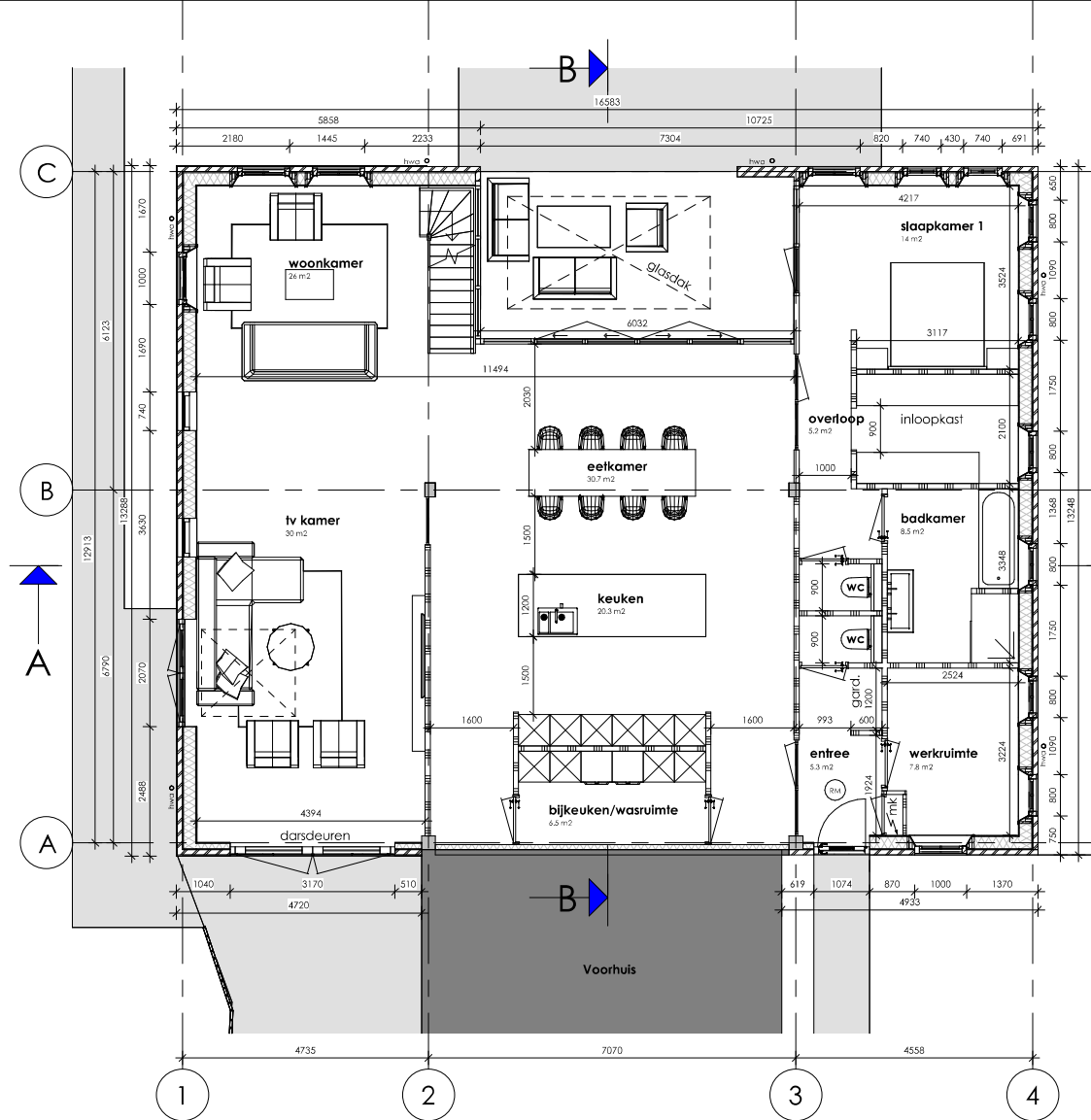
Begane grond
