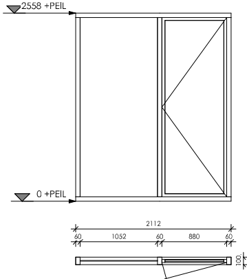
Merk G Pui met loopdeur aantal: 1
