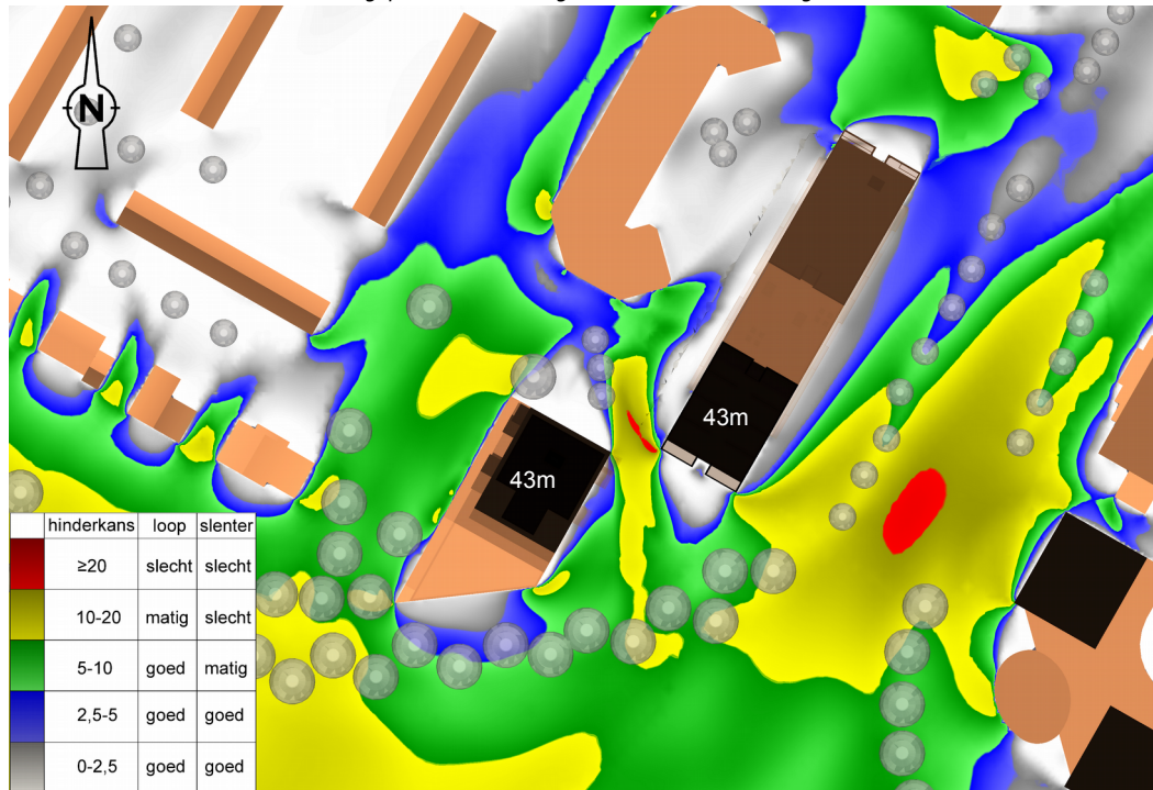
f3.2 Het te verwachten windklimaat in de geplande bebouwingssituatie, beoordeeld volgens de NEN 8100
