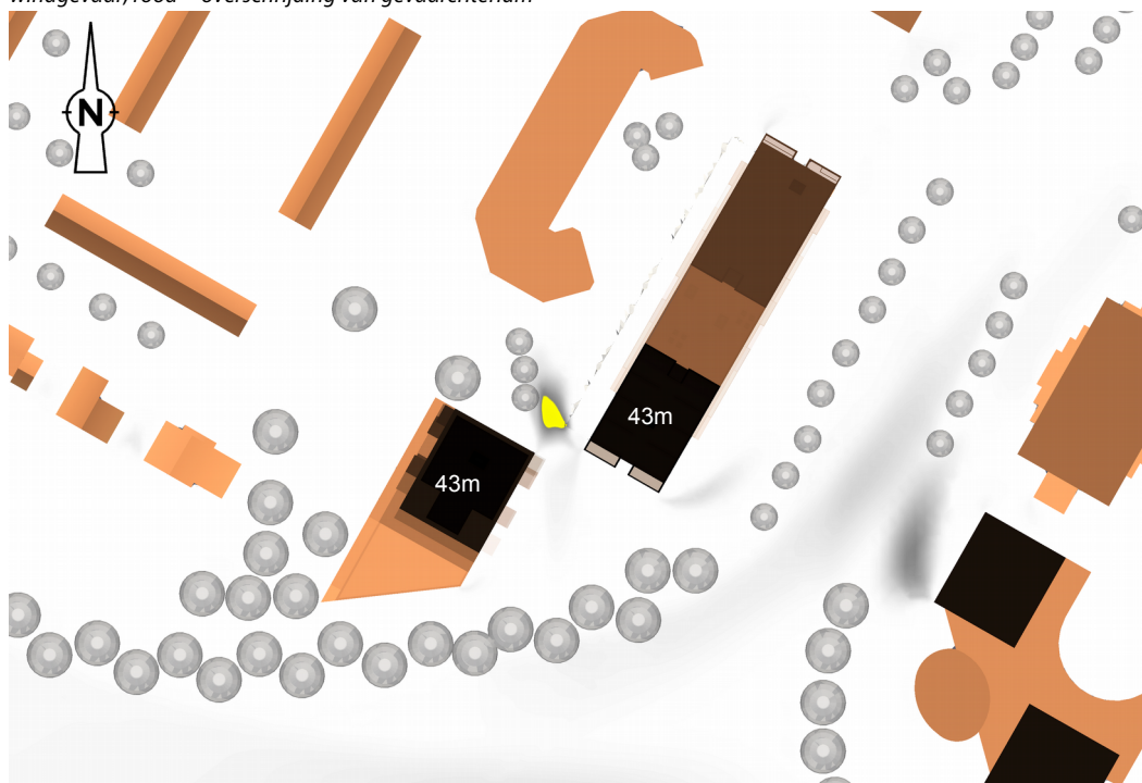
f3.3 Gevaarkans contouren, beoordeeld volgens de NEN 8100 met een drempelwaarde van 15 m/s; geel = beperkt risico op windgevaar, rood = overschrijding van gevaaercriterium
