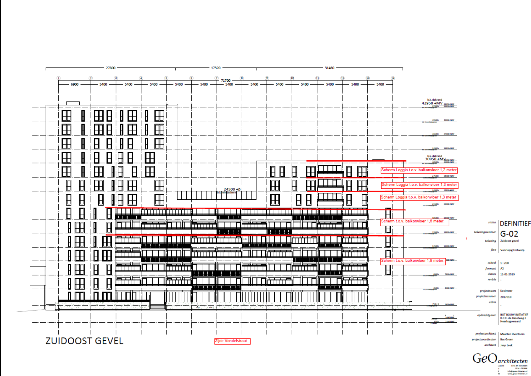
Figuur 6 per verdieping weergave minimale hoogte balkonafscherming
