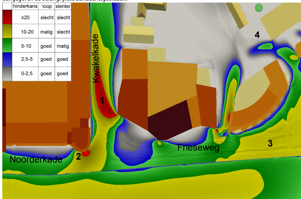
f3.3 Het te verwachten windklimaat in de geplande bestemmingplansituatie, beoordeeld volgens de NEN 8100, met daarin aangegeven de belangrijkste aandachtsgebieden.
