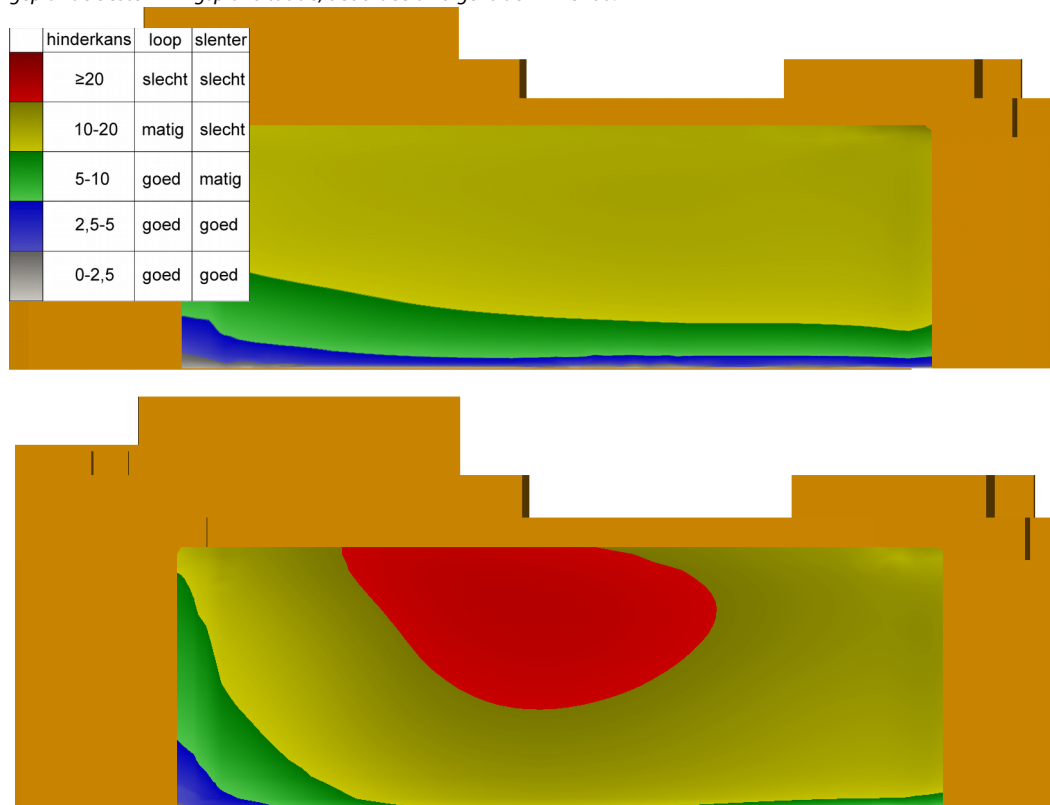
f3.4 Het te verwachten windklimaat voor de gevel van de bestaande bebouwing aan de Kwakelkade in de bestaande en de geplande bestemmingsplansituatie, beoordeeld volgens de NEN 8100.
