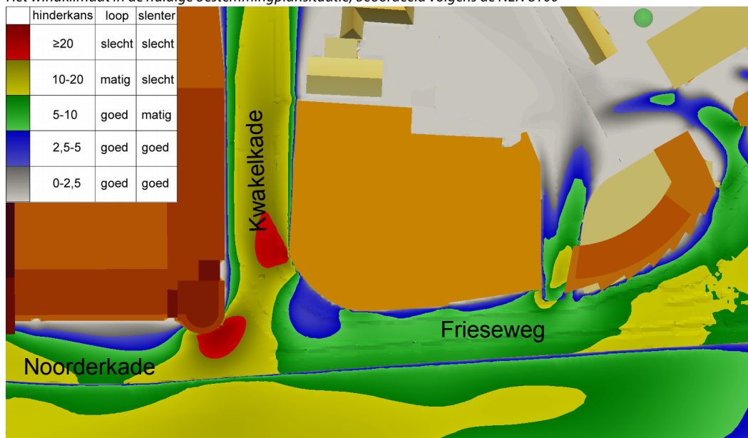
f3.2 Het windklimaat in de huidige bestemmingplansituatie, beoordeeld volgens de NEN 8100
