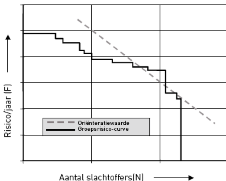
Figuur 1 Voorbeeld van een groepsrisicocurve
