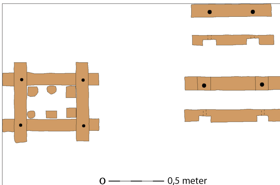
Afbeelding 8: Spoor 2C, detail van de constructie van het houtwerk (rechts de afzonderlijke delen, links een bovenaanzicht van het raamwerk met ingeheide palen).
