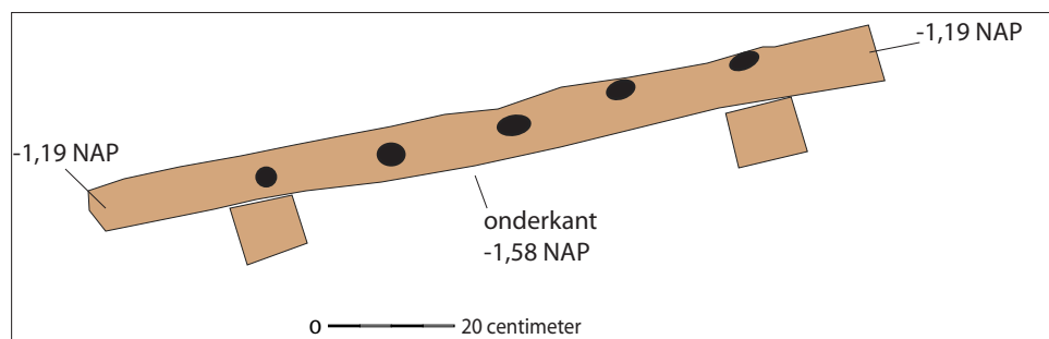
Afbeelding 4: Spoor 1A.
