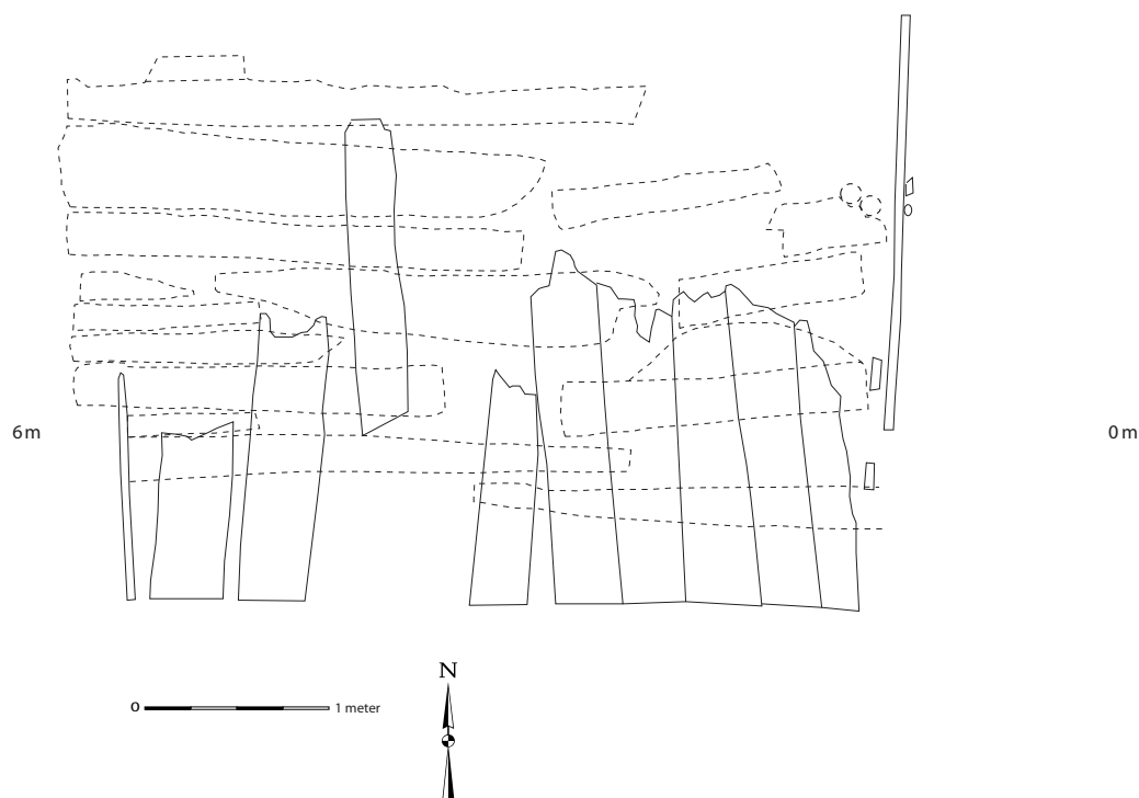
Afbeelding 16: Helling 2: De bovenliggers (doorgetrokken lijnen) en de onderliggers (gestippelde lijnen).
