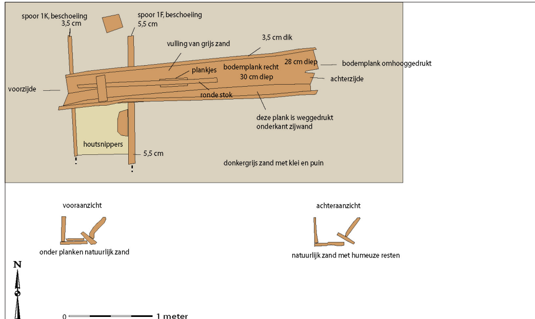
Afbeelding 6: Spoor 1E, een naaldhouten goot uit 1550-1575.
