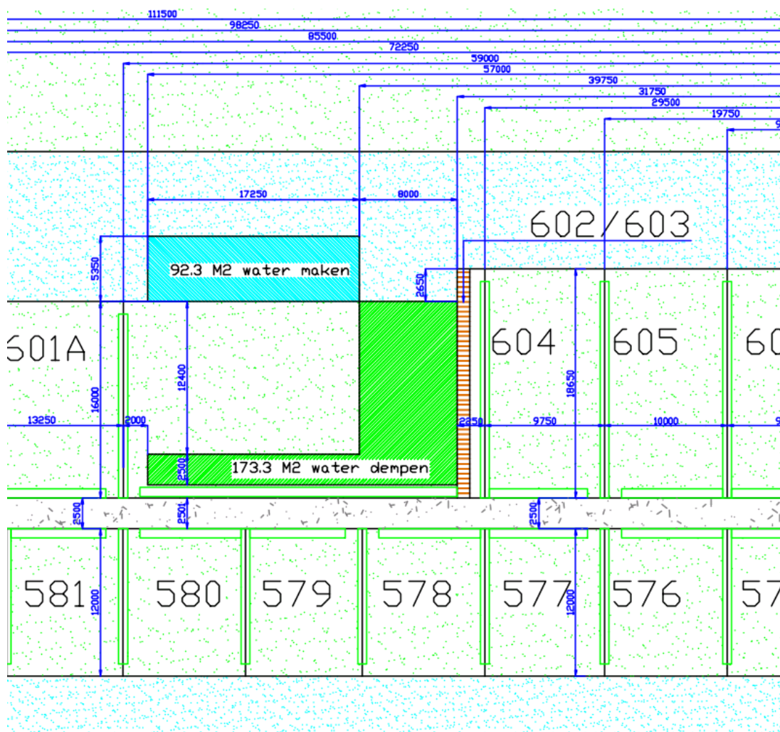
afbeelding: tekening te dempen en graven water
