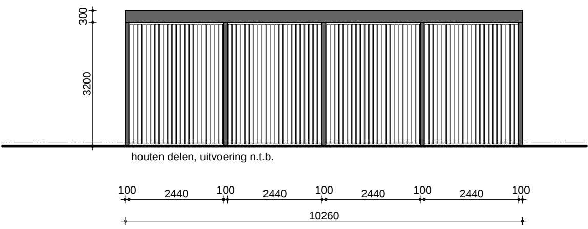
Kopse kant overkapping 3
