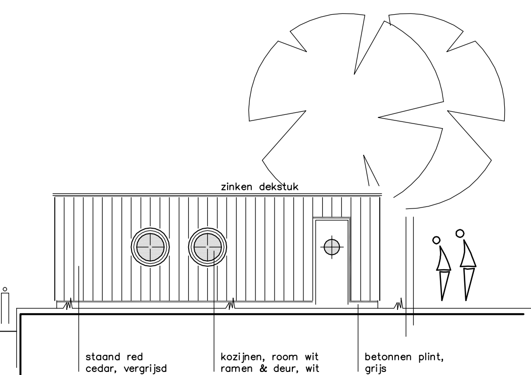
noord - westgevel
