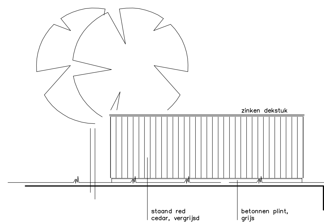
zuid - oostgevel
