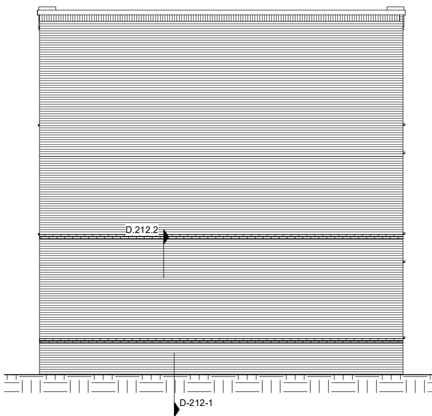
linkerzijgevel blok 7
