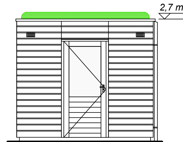
ACHTERGEVEL
