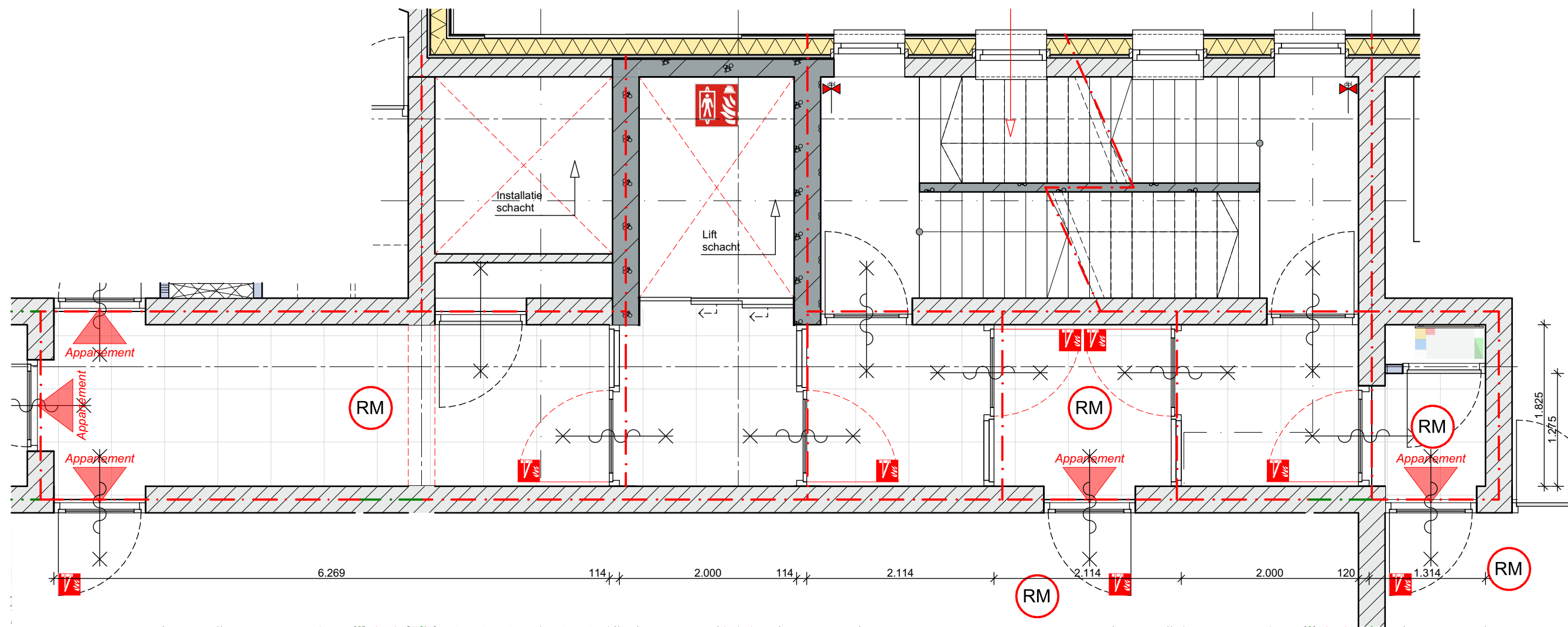
Fragment 1:50 3de t/m 5de verdieping
