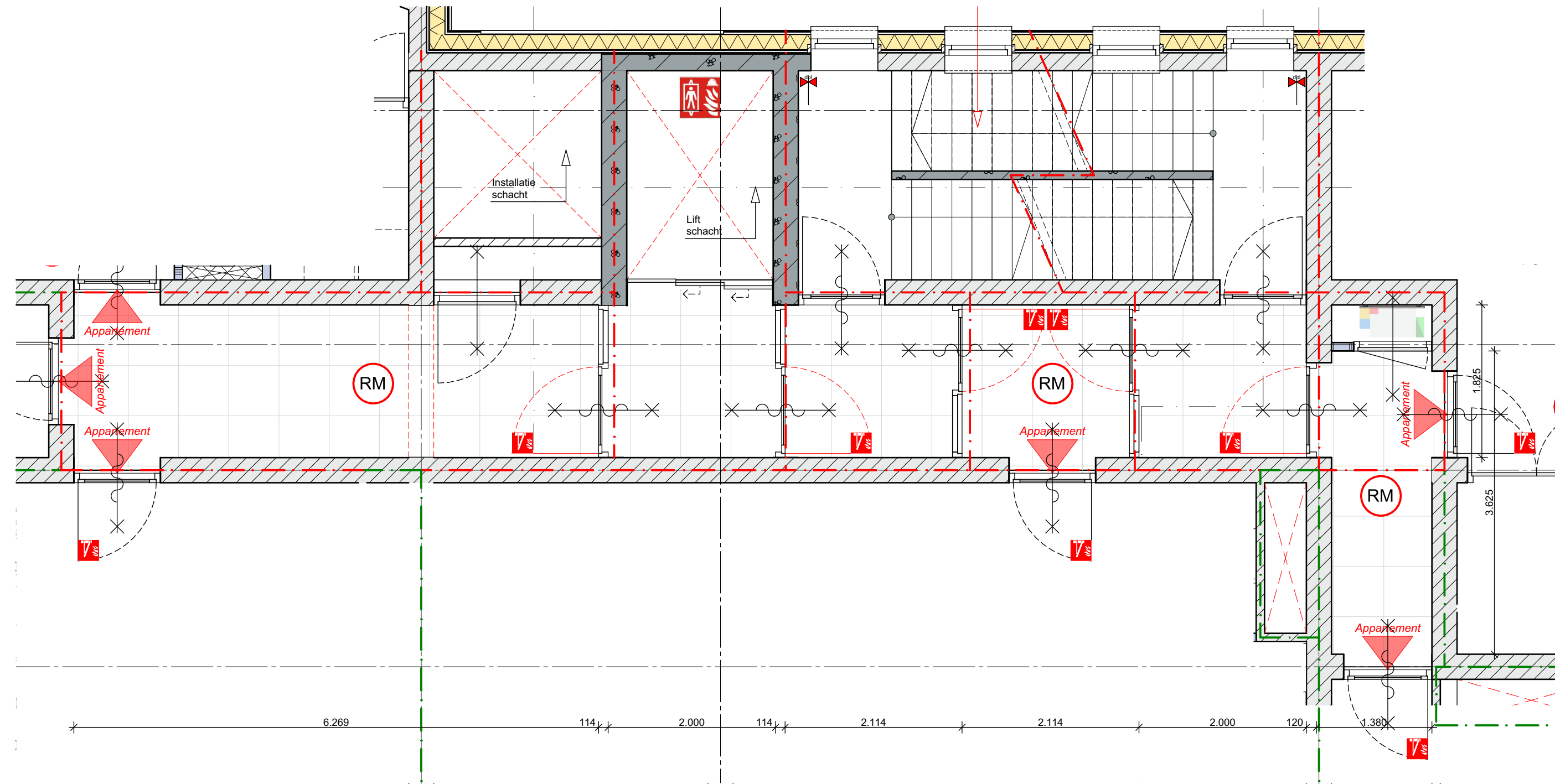
Fragment 1:50 2de verdieping
