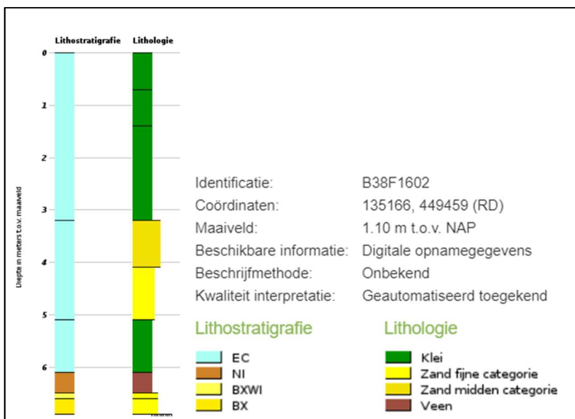
Regionale bodemopbouw (bron: Dinoloket)
