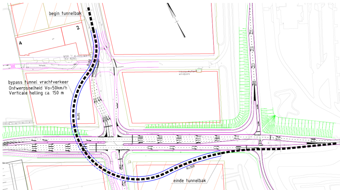
Afbeelding 4.2 Ruimtebeslag tunnel
