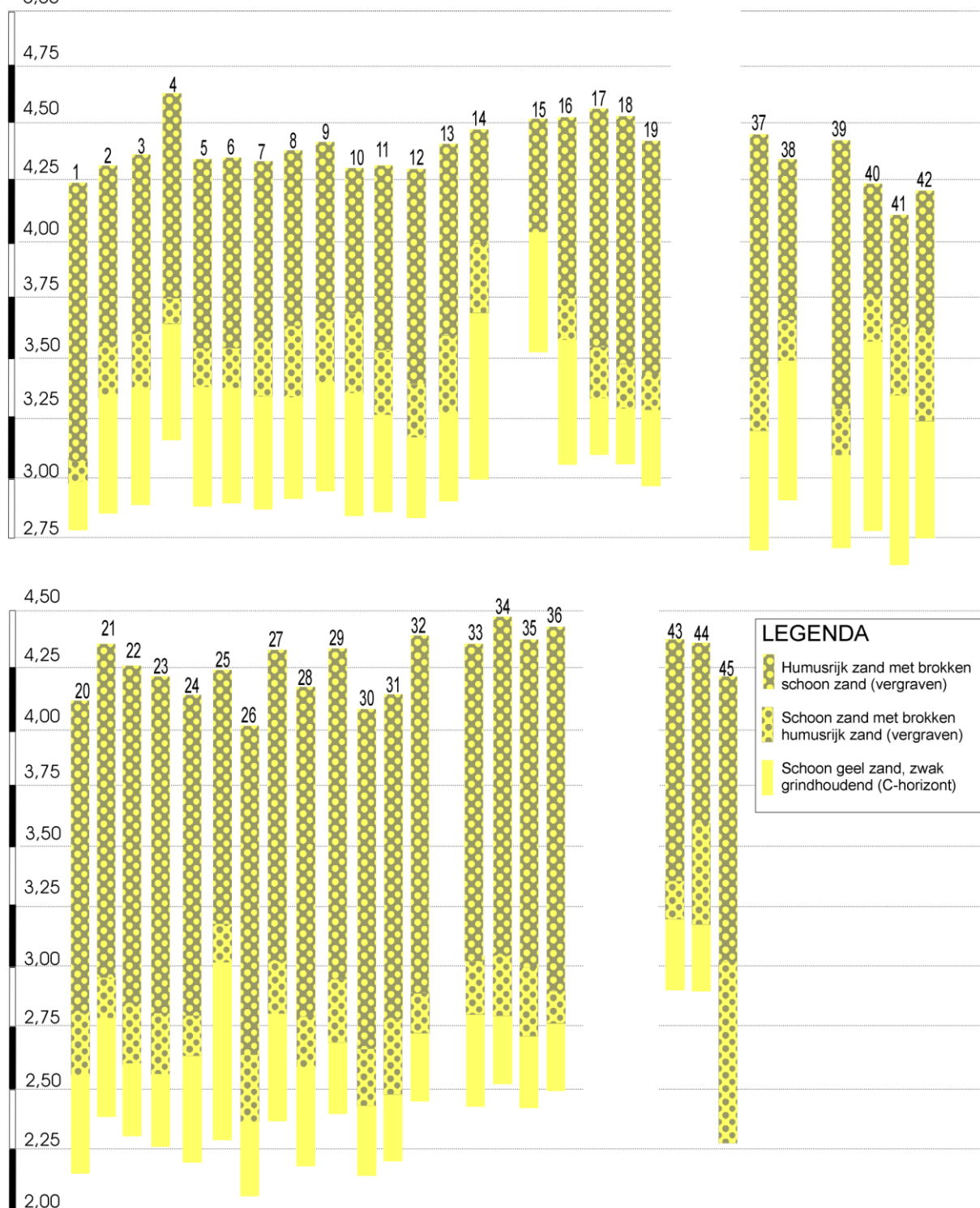
Figuur 17: Boorprofielen
