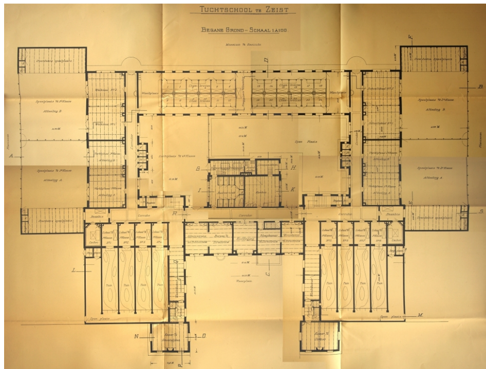
Plattegrond van de begane grond, 1904 (Herkomst: NA Den Haag)
