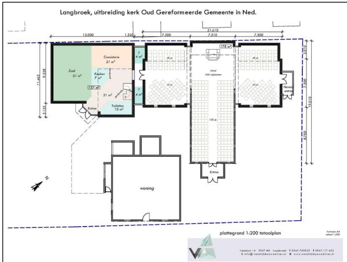
Figuur 10. Plantekening van de toekomstige na realisatie fase 2 van de voorgenomen plannen.
