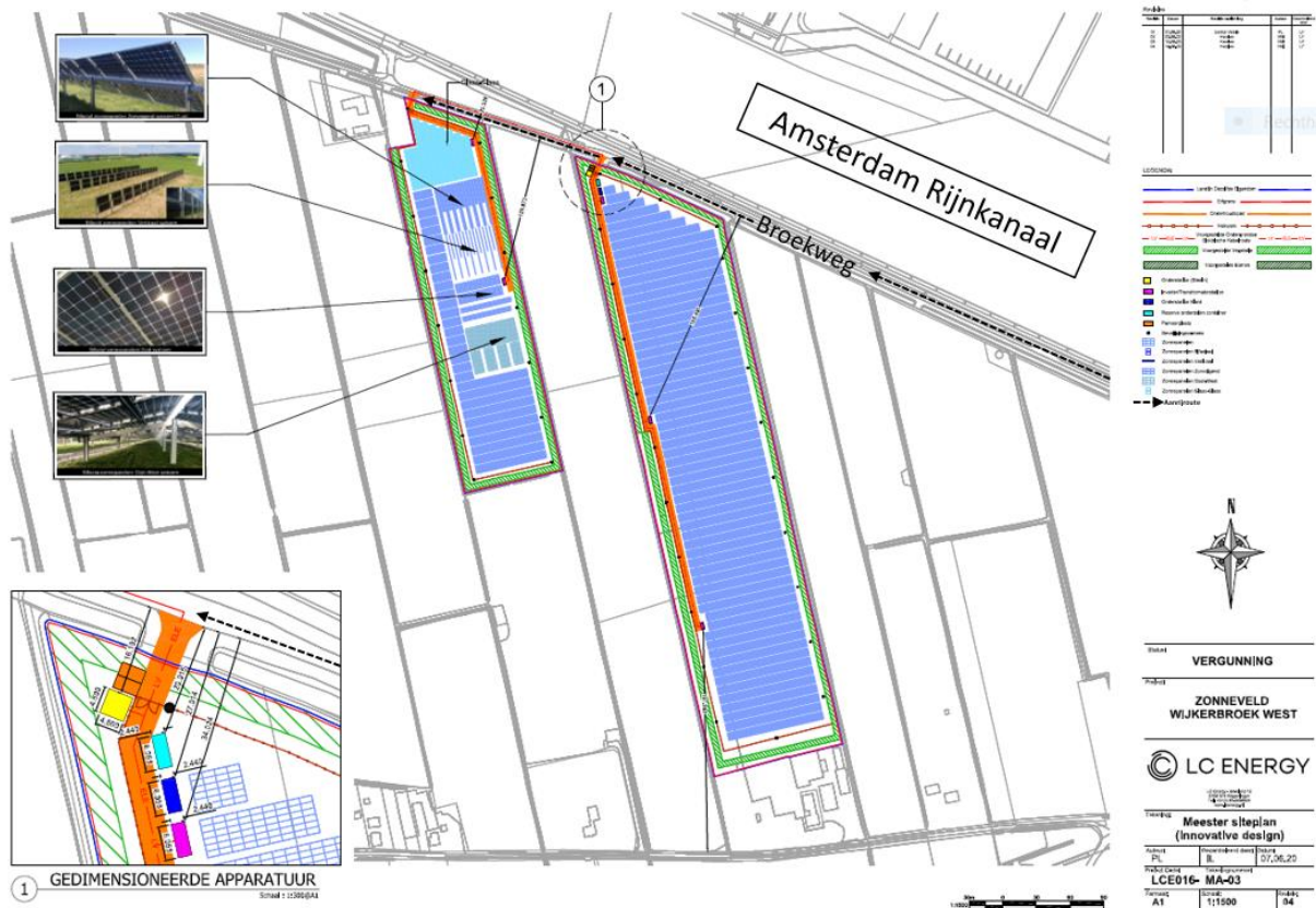
Figuur 10. Technische tekening Zonneveld Wijkerbroek West met de aanrijroute voor hulpdiensten en de andere – in de legenda – toegelichte elementen van belang.
