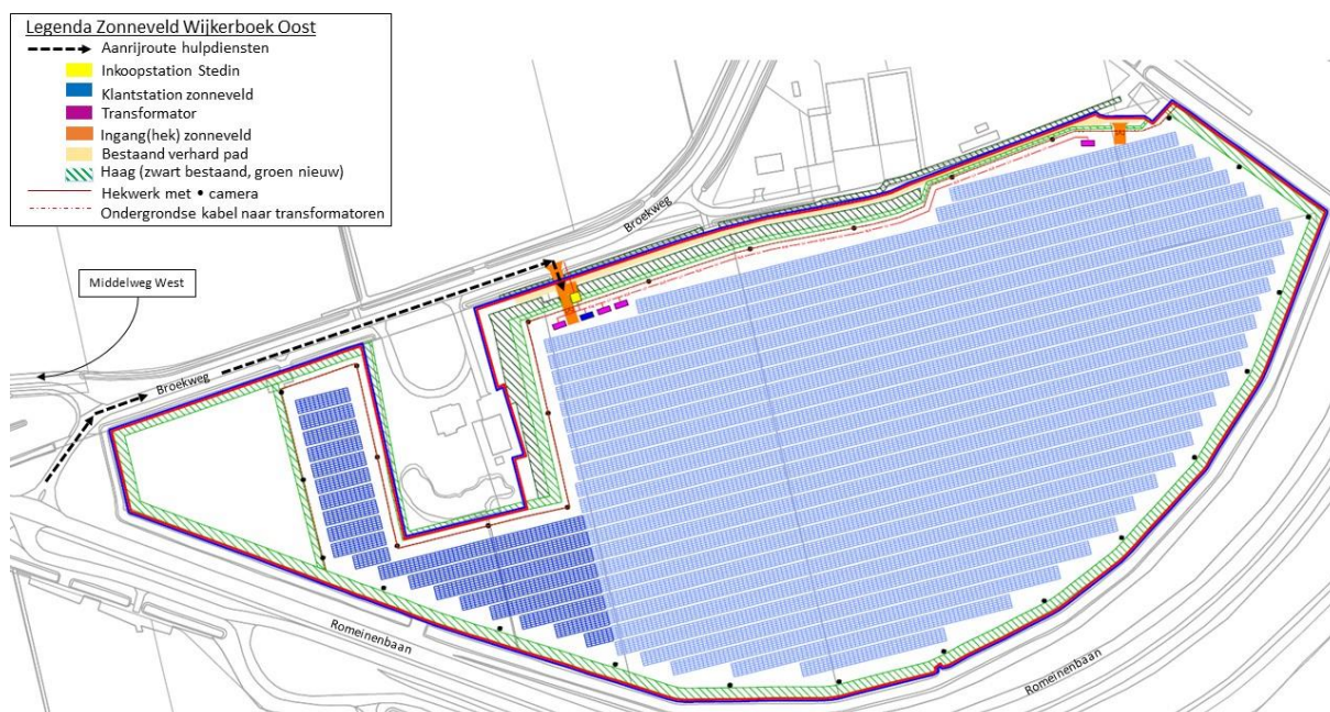
Figuur 10. Technische tekening Zonneveld Wijkerbroek Oost met de aanrijroute voor hulpdiensten en de andere – in de legenda – toegelichte elementen van belang.
