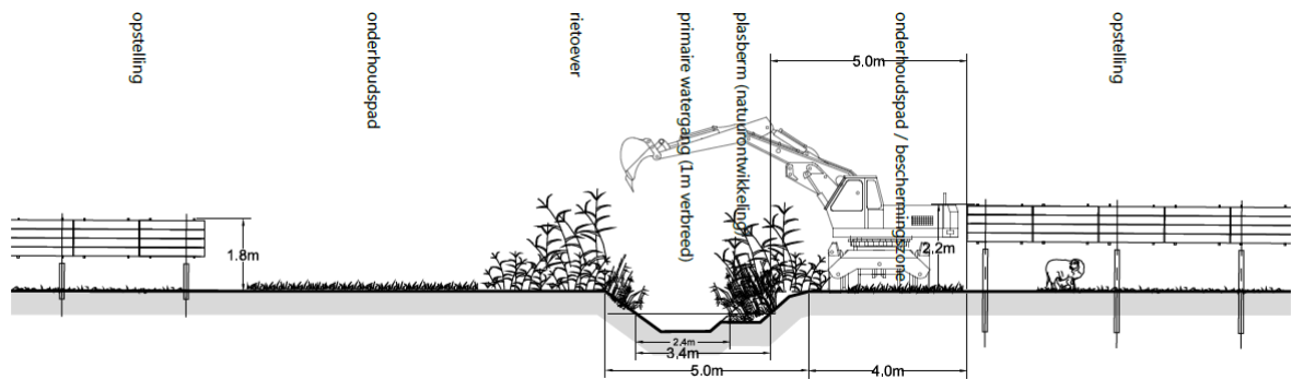
Profiel 1 schaal 1:100
