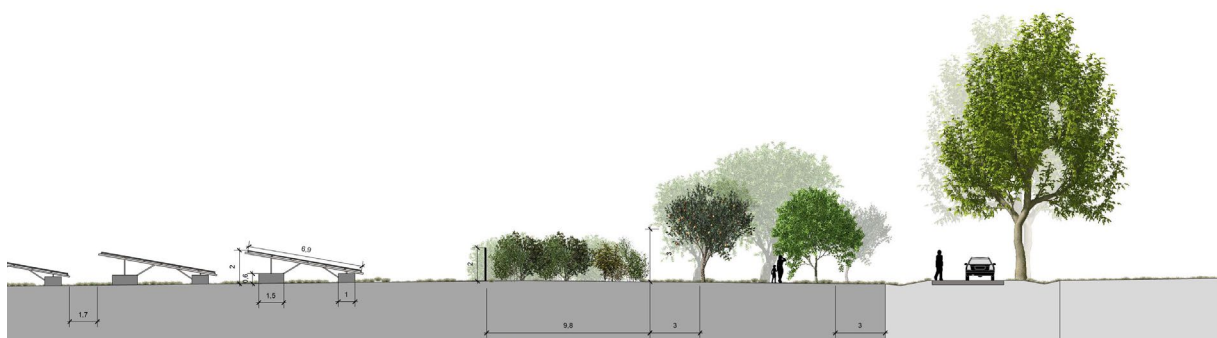
Afbeelding 22. Doorsnede A-a: watergang aan westzijde met onderhoudsroute waterschap en inpassing zonnenveld.
