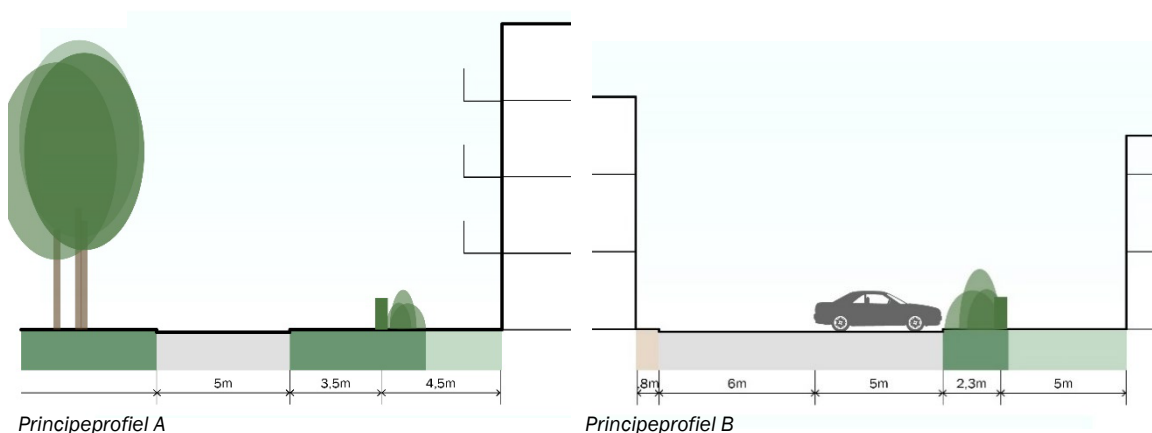
Principeprofiel A
