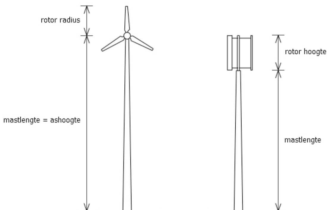
Afbeelding 2.1: de verschillen tussen het type HAT (links) en VAT (rechts).
