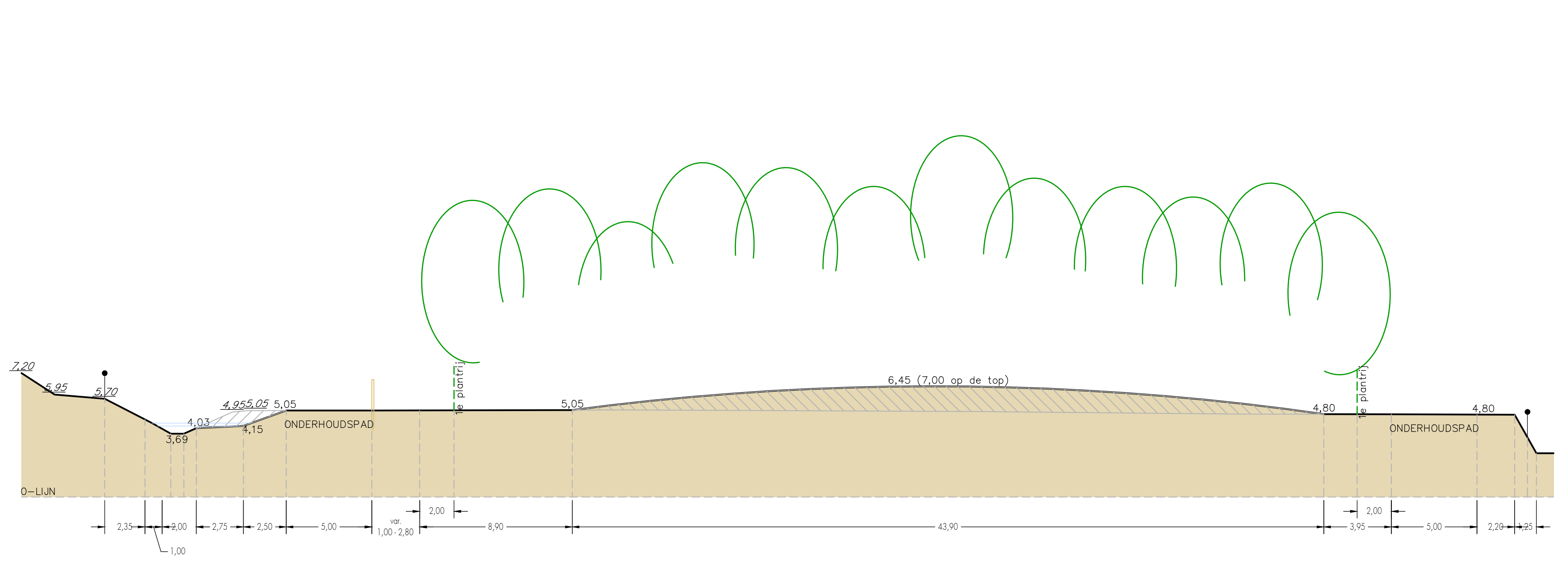
Principeprofiel B SCHAAL 1:200
