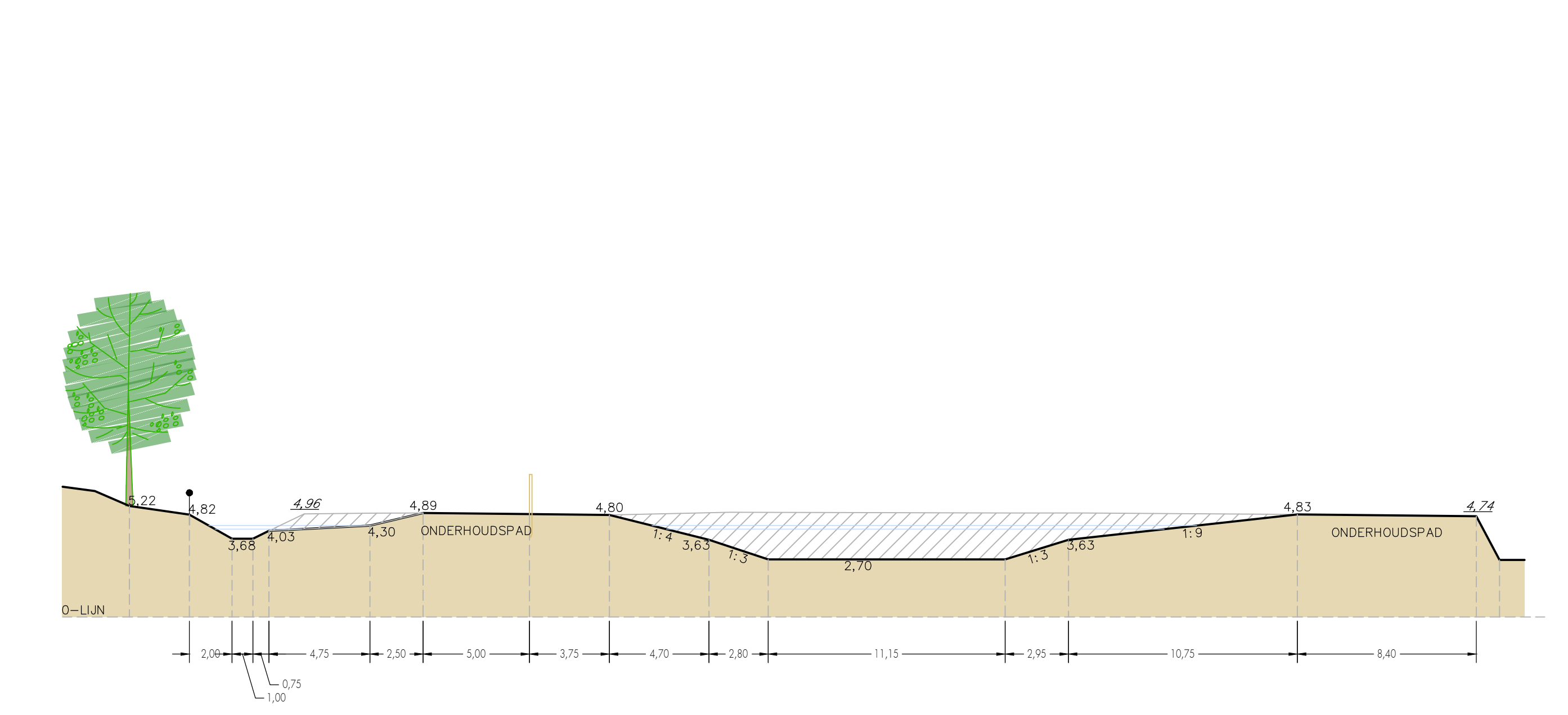
Principeprofiel A1 SCHAAL 1:200
