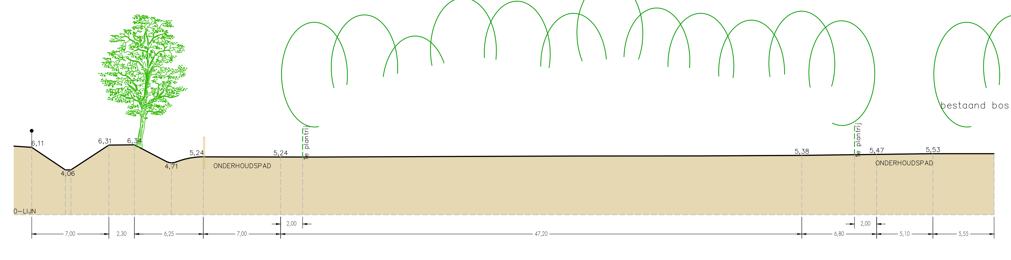
Principeprofiel C SCHAAL 1:200
