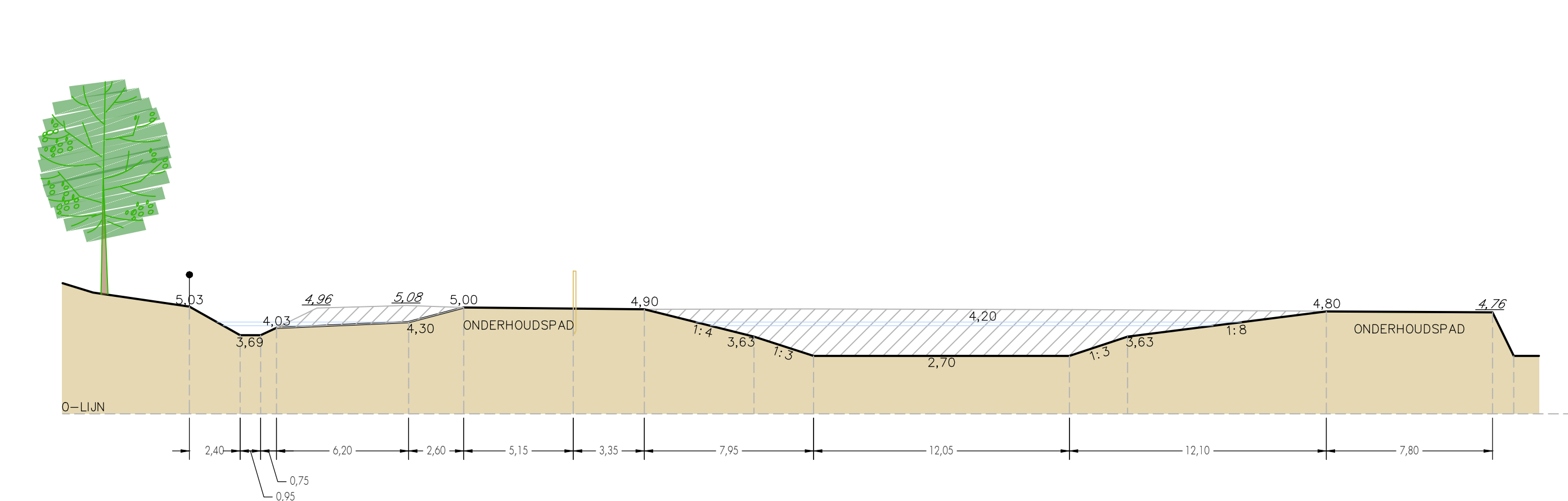
Principeprofiel A2 SCHAAL 1:200
