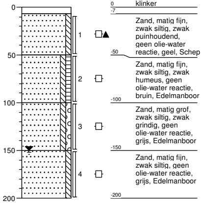
Boring: 05 boormeester J.Tibben Sleuflengte [m]: 0,30 Sleufbreedte [m]: 0,30
