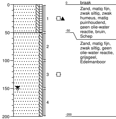
Boring: 03 boormeester J.Tibben Sleuflengte [m]: 0,30 Sleufbreedte [m]: 0,30
