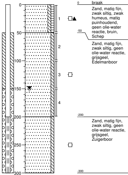
Boring: 01 boormeester J.Tibben Sleuflengte [m]: 0,30 Sleufbreedte [m]: 0,30
