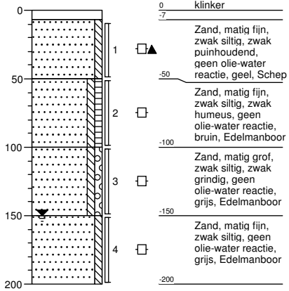
Boring: 04 boormeester J.Tibben Sleuflengte [m]: 0,30 Sleufbreedte [m]: 0,30
