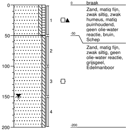
Boring: 02 boormeester J.Tibben Sleuflengte [m]: 0,30 Sleufbreedte [m]: 0,30
