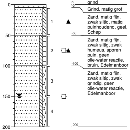
Boring: 06 boormeester J.Tibben Sleuflengte [m]: 0,30 Sleufbreedte [m]: 0,30
