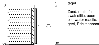
Boring: 4 boormeester j molenkamp Sleuflengte [m]: 0,00 Sleufbreedte [m]: 0,00
