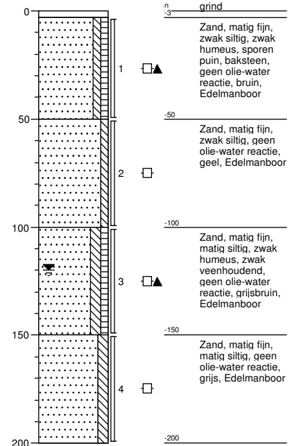
Boring: 3 boormeester j molenkamp Sleuflengte [m]: 0,00 Sleufbreedte [m]: 0,00
