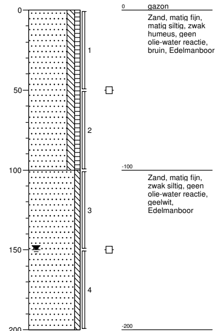
Boring: 6 boormeester j molenkamp Sleuflengte [m]: 0,00 Sleufbreedte [m]: 0,00
