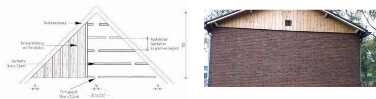
Figuur 4. Voorbeeld van gevelbetimmering die geschikt is voor vleermuizen. Bron: vleermuizenindestad.nl en checklistgroenbouwen.nl
