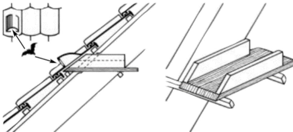
Figuur 6. Voorbeeld van een dakkast voor vleermuizen, waarbij een opening in het dak toegang biedt tot een kast aan de binnenzijde van het dakbeschot. Bron: Fledermaus Schutz im Siedlungsbereich, Deutscher Verband für Landschaftspflege.
