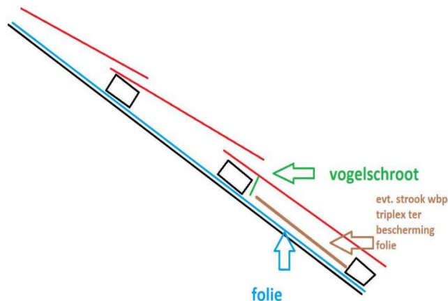
Figuur 11. Schematische tekening van het dak, waarbij het dak geschikt wordt gehouden voor huismus. Bij gebruikt vogelschroot moet dit minimaal voorbij de derde dakpan geplaatst worden., en bij voorkeur hoger.
