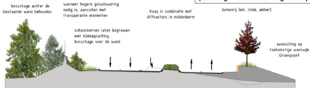
Indicatief profiel Rondweg-oost, met geluidswerende voorzieningen
