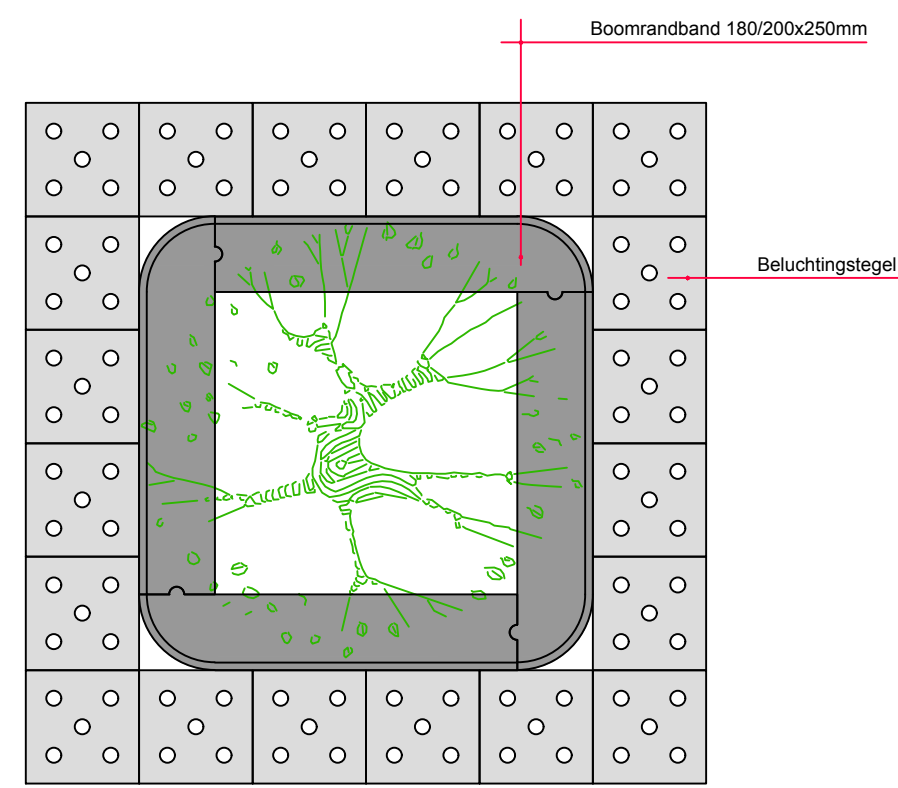
Principe Detail (schaal 1:20)
